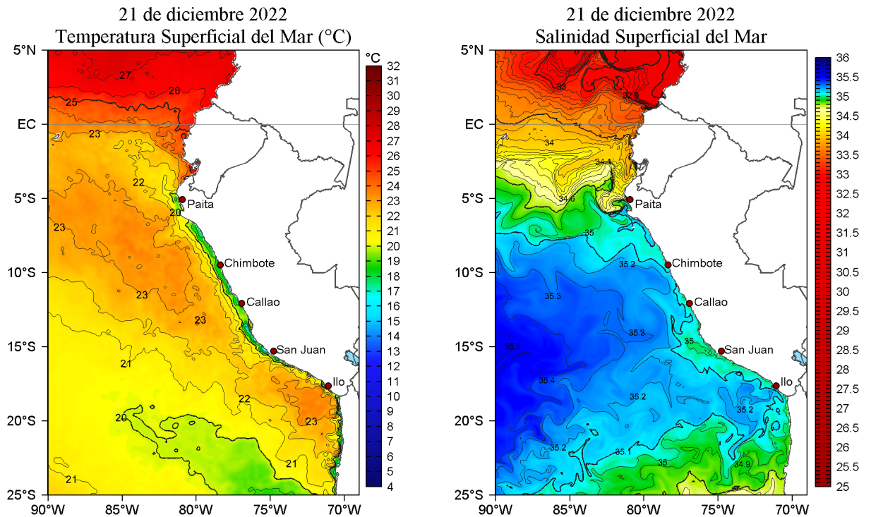
Figura 2. Temperatura superficial del mar (a la izquierda) y Salinidad superficial del mar (a la derecha) para el 21 de diciembre de 2022. Datos: OSTIA-UKMO-L4-GLOB-v2.0 (UK Met Office, 2012; Donlon et al, 2012) y Hybrid Coordinate Ocean Model v. GOFS 3.1 (HYCOM; Halliwell et al., 1998; 2000; Bleck, 2001), respectivamente.
