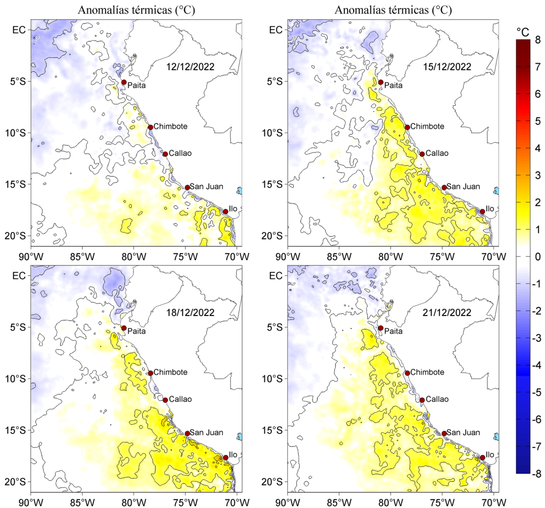
Figura 3. Anomalías de la temperatura superficial del mar (°C) para el 12, 15, 18 y 21 de diciembre de 2022. Las anomalías se calcularon respecto de la climatología para el periodo 2007-2016. Datos: OSTIA-UKMO-L4-GLOB-v2.0 (UK Met Office, 2012; Donlon et al, 2012).
