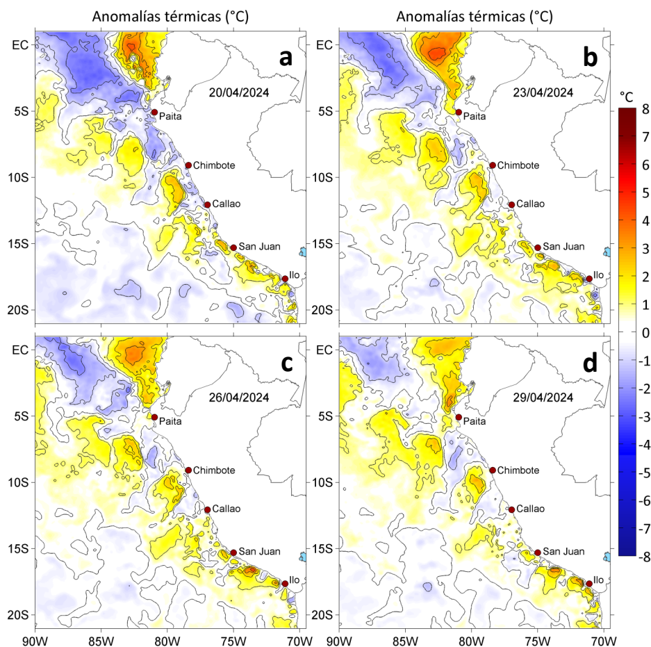
Figura 3. Anomalías de la temperatura superficial del mar ( ^{\circ}\text{C} ) para el a) 20, b) 23, c) 26 y d) 29 de abril de 2024. Las anomalías se calcularon respecto de la climatología para el periodo 1991-2020. Datos: OSTIA-UKMO-L4-GLOB-v2.0 (UK Met Office, 2012; Donlon et al, 2012).
