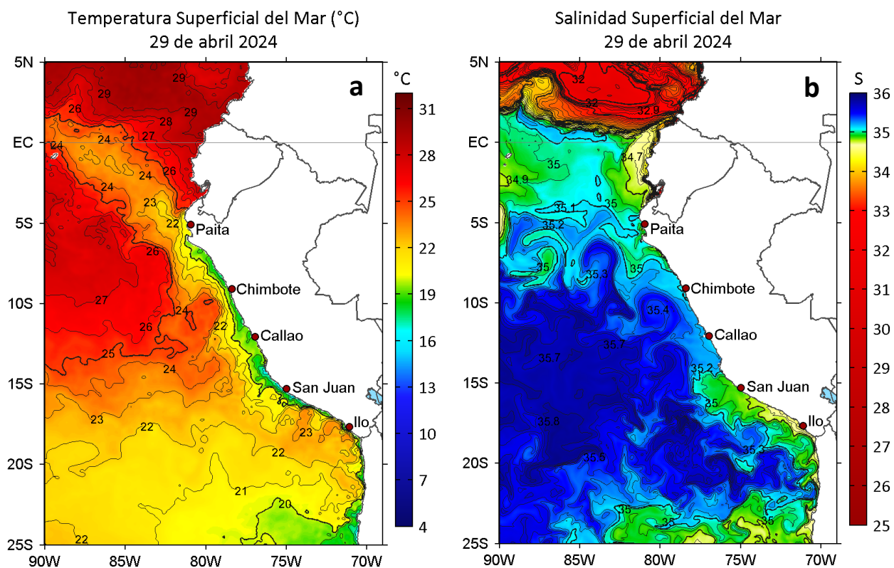
Figura 2. a) Temperatura superficial del mar ( ^{\circ}\text{C} ) y b) Salinidad superficial del mar para el 29 de abril de 2024. Datos: OSTIA-UKMO-L4-GLOB-v2.0 (UK Met Office, 2012; Donlon et al, 2012) y del GLOBAL_ANALYSISFORECAST_PHY_001_024 (Lellouche, J. M. et al, 2013), respectivamente.
