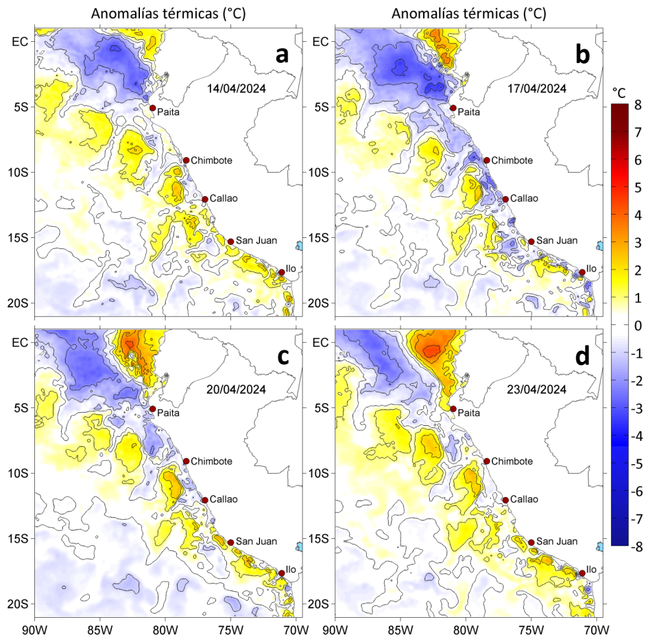
Figura 3. Anomalías de la temperatura superficial del mar ( ^{\circ}\text{C} ) para el a) 14, b) 17, c) 20 y d) 23 de abril de 2024. Las anomalías se calcularon respecto de la climatología para el periodo 1991-2020. Datos: OSTIA-UKMO-L4-GLOB-v2.0 (UK Met Office, 2012; Donlon et al, 2012).
