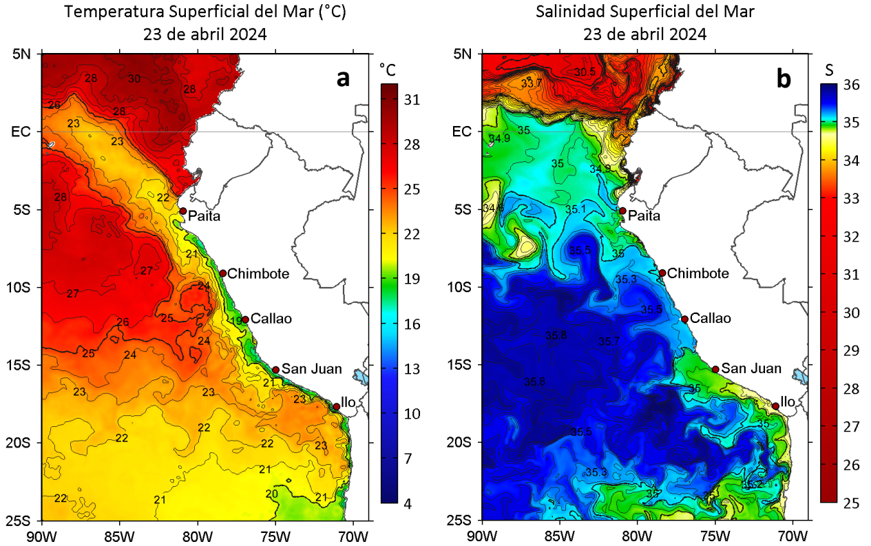
Figura 2. a) Temperatura superficial del mar ( ^{\circ}\text{C} ) y b) Salinidad superficial del mar para el 23 de abril de 2024. Datos: OSTIA-UKMO-L4-GLOB-v2.0 (UK Met Office, 2012; Donlon et al, 2012) y del GLOBAL_ANALYSISFORECAST_PHY_001_024 (Lellouche, J. M. et al, 2013), respectivamente.
