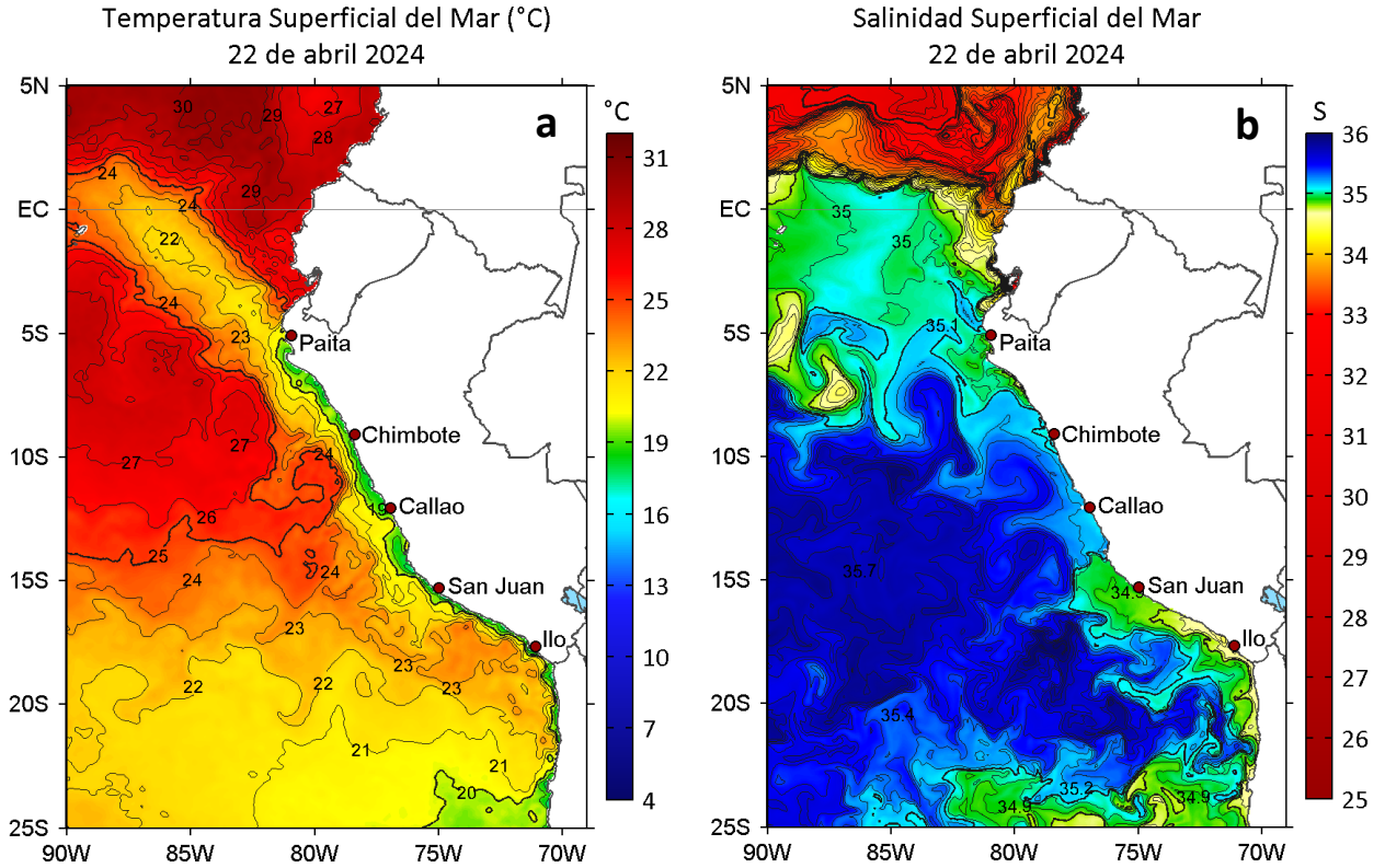
Figura 2. a) Temperatura superficial del mar (°C) y b) Salinidad superficial del mar para el 22 de abril de 2024. Datos: OSTIA-UKMO-L4-GLOB-v2.0 (UK Met Office, 2012; Donlon et al, 2012) y del GLOBAL_ANALYSISFORECAST_PHY_001_024 (Lellouche, J. M. et al, 2013), respectivamente.
