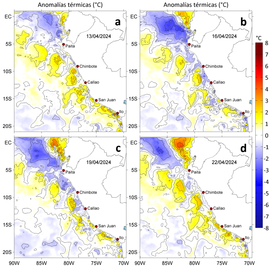
Figura 3. Anomalías de la temperatura superficial del mar (°C) para el a) 13, b) 16, c) 19 y d) 22 de abril de 2024. Las anomalías se calcularon respecto de la climatología para el periodo 1991-2020. Datos: OSTIA-UKMO-L4-GLOB-v2.0 (UK Met Office, 2012; Donlon et al, 2012).
