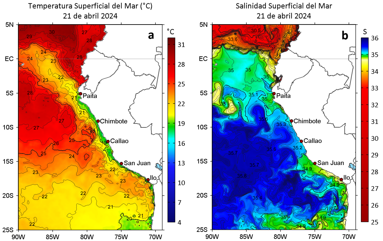
Figura 2. a) Temperatura superficial del mar ( ^{\circ}\text{C} ) y b) Salinidad superficial del mar para el 21 de abril de 2024. Datos: OSTIA-UKMO-L4-GLOB-v2.0 (UK Met Office, 2012; Donlon et al, 2012) y del GLOBAL_ANALYSISFORECAST_PHY_001_024 (Lellouche, J. M. et al, 2013), respectivamente.
