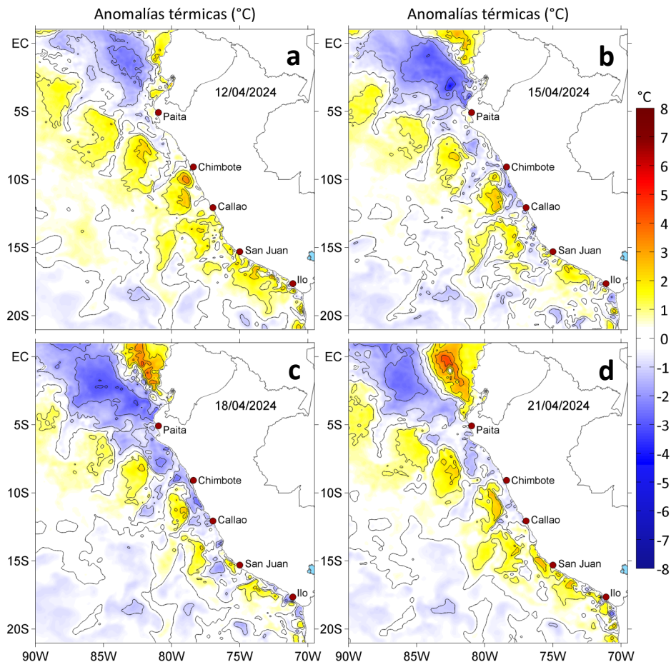
Figura 3. Anomalías de la temperatura superficial del mar ( ^{\circ}\text{C} ) para el a) 12, b) 15, c) 18 y d) 21 de abril de 2024. Las anomalías se calcularon respecto de la climatología para el periodo 1991-2020. Datos: OSTIA-UKMO-L4-GLOB-v2.0 (UK Met Office, 2012; Donlon et al, 2012).
