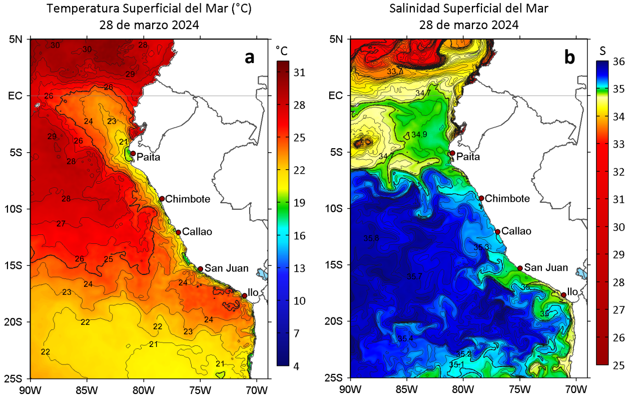
Figura 2. a) Temperatura superficial del mar ( ^{\circ}\text{C} ) y b) Salinidad superficial del mar para el 28 de marzo de 2024. Datos: OSTIA-UKMO-L4-GLOB-v2.0 (UK Met Office, 2012; Donlon et al, 2012) y del GLOBAL_ANALYSISFORECAST_PHY_001_024 (Lellouche, J. M. et al, 2013), respectivamente.
