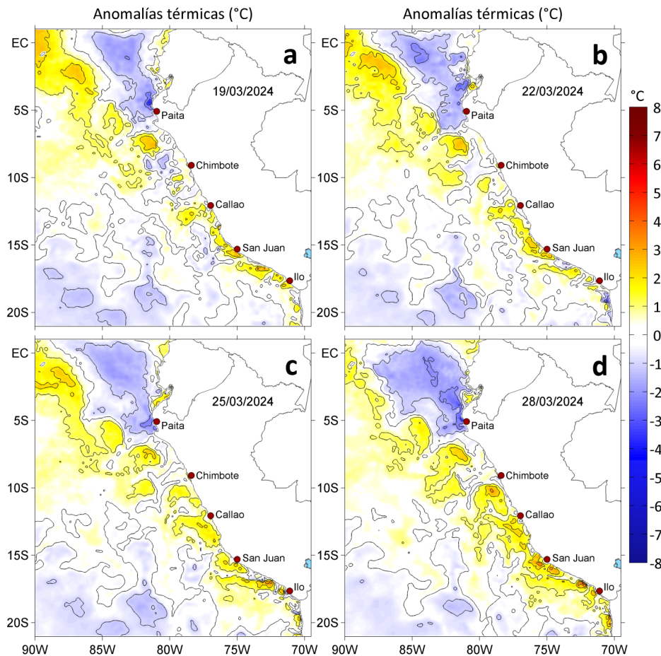
Figura 3. Anomalías de la temperatura superficial del mar ( ^{\circ}\text{C} ) para el a) 19, b) 22, c) 25 y d) 28 de marzo de 2024. Las anomalías se calcularon respecto de la climatología para el periodo 1991-2020. Datos: OSTIA-UKMO-L4-GLOB-v2.0 (UK Met Office, 2012; Donlon et al, 2012).
