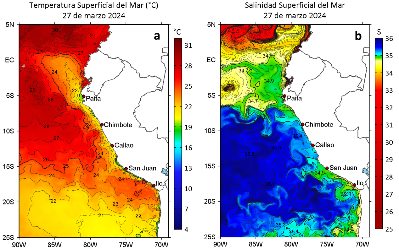
Figura 2. a) Temperatura superficial del mar (°C) y b) Salinidad superficial del mar para el 27 de marzo de 2024. Datos: OSTIA-UKMO-L4-GLOB-v2.0 (UK Met Office, 2012; Donlon et al, 2012) y del GLOBAL_ANALYSISFORECAST_PHY_001_024 (Lellouche, J. M. et al, 2013), respectivamente.
