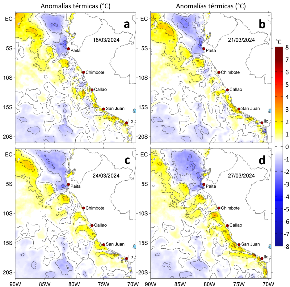
Figura 3. Anomalías de la temperatura superficial del mar (°C) para el a) 18, b) 21, c) 24 y d) 27 de marzo de 2024. Las anomalías se calcularon respecto de la climatología para el periodo 1991-2020. Datos: OSTIA-UKMO-L4-GLOB-v2.0 (UK Met Office, 2012; Donlon et al, 2012).
