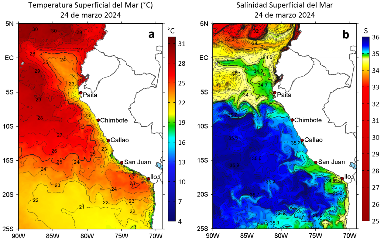
Figura 2. a) Temperatura superficial del mar (°C) y b) Salinidad superficial del mar para el 24 de marzo de 2024. Datos: OSTIA-UKMO-L4-GLOB-v2.0 (UK Met Office, 2012; Donlon et al, 2012) y del GLOBAL_ANALYSISFORECAST_PHY_001_024 (Lellouche, J. M. et al, 2013), respectivamente.
