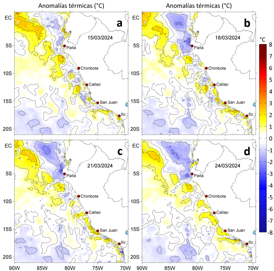
Figura 3. Anomalías de la temperatura superficial del mar (°C) para el a) 15, b) 18, c) 21 y d) 24 de marzo de 2024. Las anomalías se calcularon respecto de la climatología para el periodo 1991-2020. Datos: OSTIA-UKMO-L4-GLOB-v2.0 (UK Met Office, 2012; Donlon et al, 2012).
