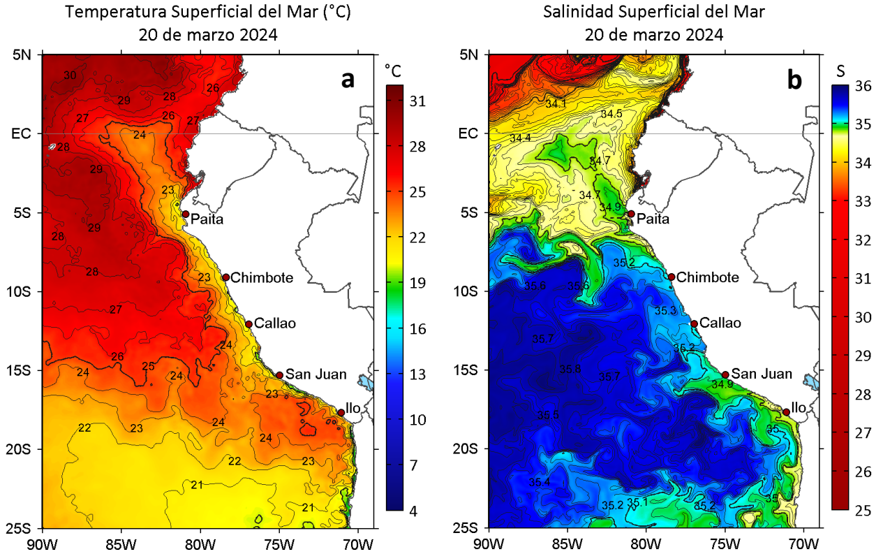
Figura 2. a) Temperatura superficial del mar ( ^{\circ}\text{C} ) y b) Salinidad superficial del mar para el 20 de marzo de 2024. Datos: OSTIA-UKMO-L4-GLOB-v2.0 (UK Met Office, 2012; Donlon et al, 2012) y del GLOBAL_ANALYSISFORECAST_PHY_001_024 (Lellouche, J. M. et al, 2013), respectivamente.
