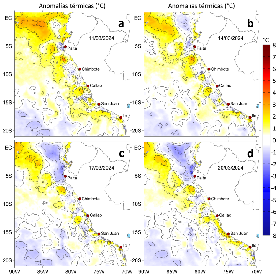
Figura 3. Anomalías de la temperatura superficial del mar ( ^{\circ}\text{C} ) para el a) 11, b) 14, c) 17 y d) 20 de marzo de 2024. Las anomalías se calcularon respecto de la climatología para el periodo 1991-2020. Datos: OSTIA-UKMO-L4-GLOB-v2.0 (UK Met Office, 2012; Donlon et al, 2012).
