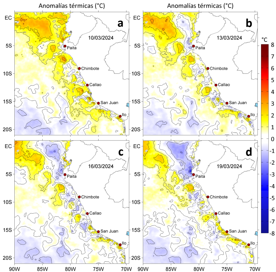
Figura 3. Anomalías de la temperatura superficial del mar ( ^{\circ}\text{C} ) para el a) 10, b) 13, c) 16 y d) 19 de marzo de 2024. Las anomalías se calcularon respecto de la climatología para el periodo 1991-2020. Datos: OSTIA-UKMO-L4-GLOB-v2.0 (UK Met Office, 2012; Donlon et al, 2012).
