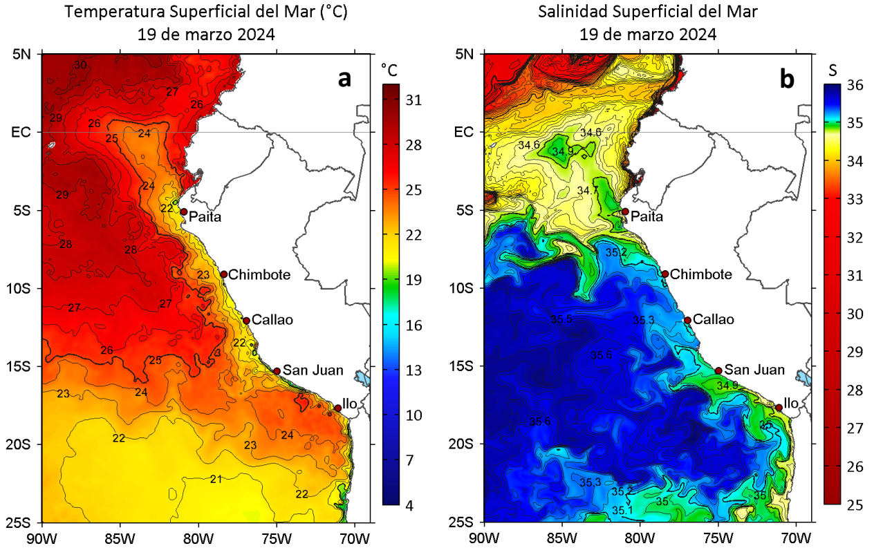
Figura 2. a) Temperatura superficial del mar ( ^{\circ}\text{C} ) y b) Salinidad superficial del mar para el 19 de marzo de 2024. Datos: OSTIA-UKMO-L4-GLOB-v2.0 (UK Met Office, 2012; Donlon et al, 2012) y del GLOBAL_ANALYSISFORECAST_PHY_001_024 (Lellouche, J. M. et al, 2013), respectivamente.
