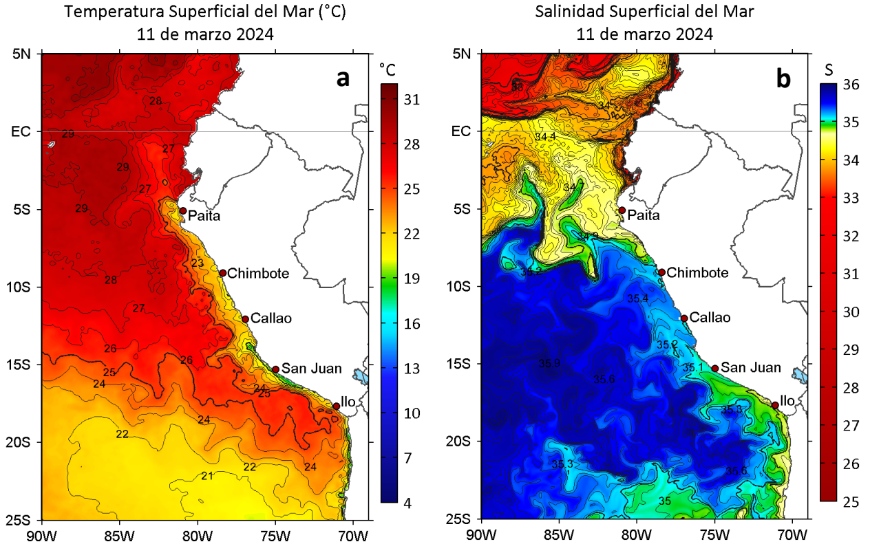
Figura 2. a) Temperatura superficial del mar ( ^{\circ}\text{C} ) y b) Salinidad superficial del mar para el 11 de marzo de 2024. Datos: OSTIA-UKMO-L4-GLOB-v2.0 (UK Met Office, 2012; Donlon et al, 2012) y del GLOBAL_ANALYSISFORECAST_PHY_001_024 (Lellouche, J. M. et al, 2013), respectivamente.
