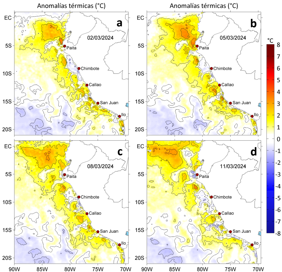
Figura 3. Anomalías de la temperatura superficial del mar ( ^{\circ}\text{C} ) para el a) 02, b) 05, c) 08 y d) 11 de marzo de 2024. Las anomalías se calcularon respecto de la climatología para el periodo 1991-2020. Datos: OSTIA-UKMO-L4-GLOB-v2.0 (UK Met Office, 2012; Donlon et al, 2012).
