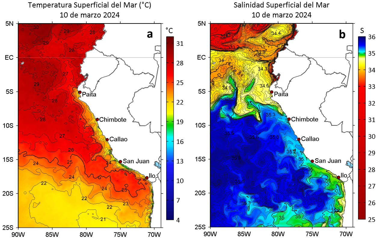
Figura 2. a) Temperatura superficial del mar (°C) y b) Salinidad superficial del mar para el 10 de marzo de 2024. Datos: OSTIA-UKMO-L4-GLOB-v2.0 (UK Met Office, 2012; Donlon et al, 2012) y del GLOBAL_ANALYSISFORECAST_PHY_001_024 (Lellouche, J. M. et al, 2013), respectivamente.
