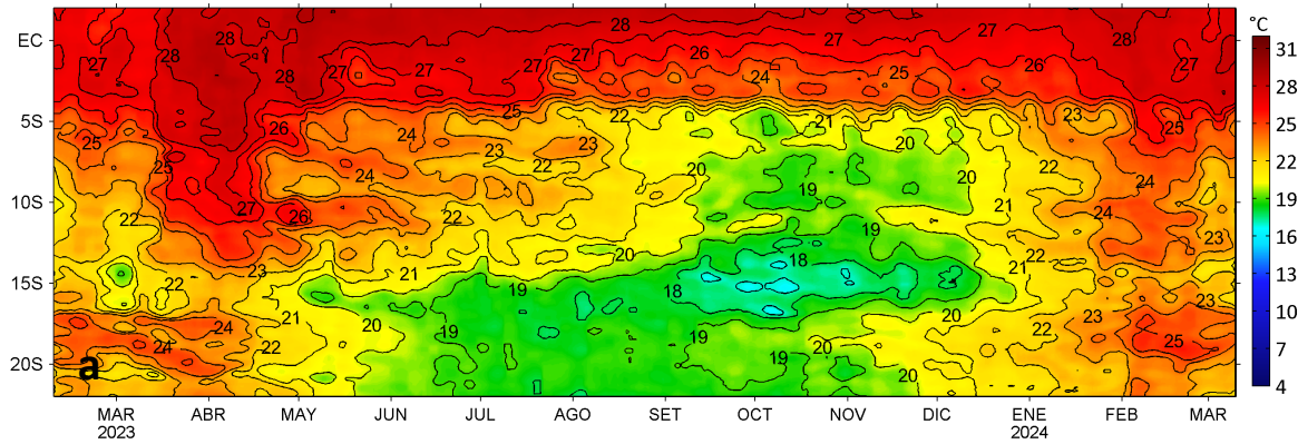
Anomalías de la Temperatura Superficial del mar (°C), franja costera de 60 mn 08 de febrero 2023 - 10 de marzo 2024
