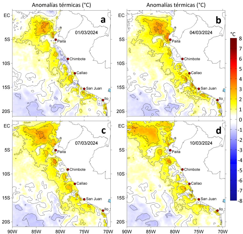
Figura 3. Anomalías de la temperatura superficial del mar (°C) para el a) 01, b) 04, c) 07 y d) 10 de marzo de 2024. Las anomalías se calcularon respecto de la climatología para el periodo 1991-2020. Datos: OSTIA-UKMO-L4-GLOB-v2.0 (UK Met Office, 2012; Donlon et al, 2012).
