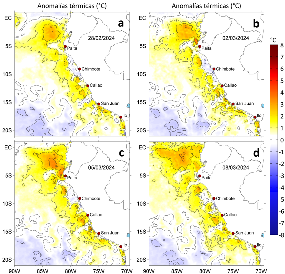
Figura 3. Anomalías de la temperatura superficial del mar ( ^{\circ}\text{C} ) para el a) 28 de febrero, b) 02, c) 05 y d) 08 de marzo de 2024. Las anomalías se calcularon respecto de la climatología para el periodo 1991-2020. Datos: OSTIA-UKMO-L4-GLOB-v2.0 (UK Met Office, 2012; Donlon et al, 2012).
