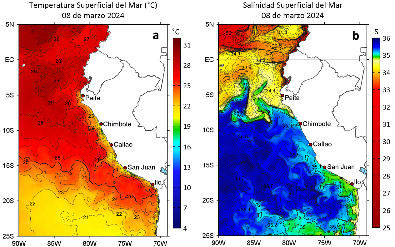
Figura 2. a) Temperatura superficial del mar ( ^{\circ}\text{C} ) y b) Salinidad superficial del mar para el 08 de marzo de 2024. Datos: OSTIA-UKMO-L4-GLOB-v2.0 (UK Met Office, 2012; Donlon et al, 2012) y del GLOBAL_ANALYSISFORECAST_PHY_001_024 (Lellouche, J. M. et al, 2013), respectivamente.
