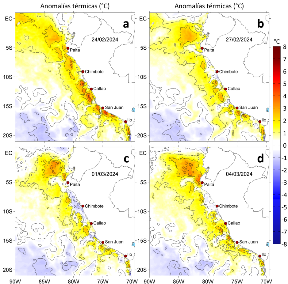
Figura 3. Anomalías de la temperatura superficial del mar ( ^{\circ}\text{C} ) para el a) 24 y b) 27 de febrero, así como para el c) 01 y d) 04 de marzo de 2024. Las anomalías se calcularon respecto de la climatología para el periodo 1991-2020. Datos: OSTIA-UKMO-L4-GLOB-v2.0 (UK Met Office, 2012; Donlon et al, 2012).
