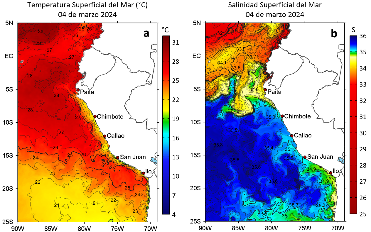
Figura 2. a) Temperatura superficial del mar ( ^{\circ}\text{C} ) y b) Salinidad superficial del mar para el 04 de marzo de 2024. Datos: OSTIA-UKMO-L4-GLOB-v2.0 (UK Met Office, 2012; Donlon et al, 2012) y del GLOBAL_ANALYSISFORECAST_PHY_001_024 (Lellouche, J. M. et al, 2013), respectivamente.
