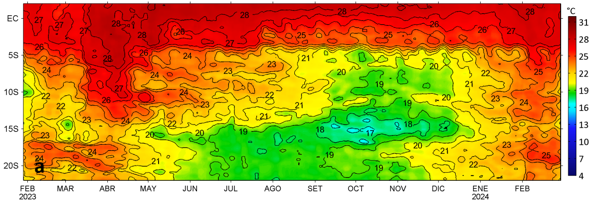
Anomalías de la Temperatura Superficial del mar (°C), franja costera de 60 mn 29 de enero 2023 - 29 de febrero 2024
