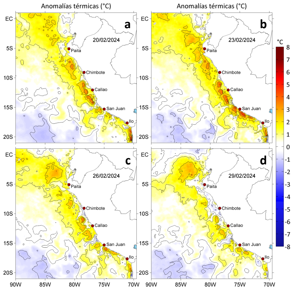
Figura 3. Anomalías de la temperatura superficial del mar ( ^{\circ}\text{C} ) para el a) 20, b) 23, c) 26 y d) 29 de febrero de 2024. Las anomalías se calcularon respecto de la climatología para el periodo 1991-2020. Datos: OSTIA-UKMO-L4-GLOB-v2.0 (UK Met Office, 2012; Donlon et al, 2012).
