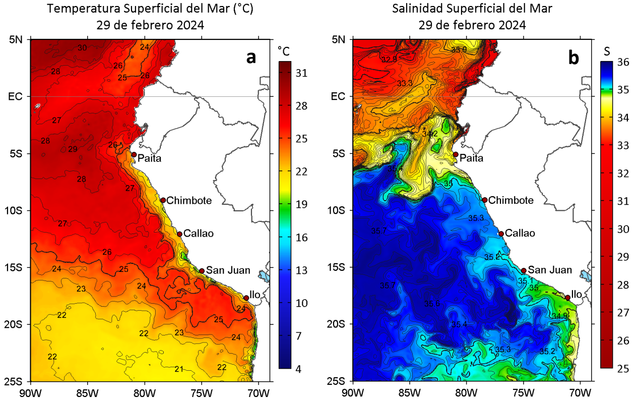
Figura 2. a) Temperatura superficial del mar ( ^{\circ}\text{C} ) y b) Salinidad superficial del mar para el 29 de febrero de 2024. Datos: OSTIA-UKMO-L4-GLOB-v2.0 (UK Met Office, 2012; Donlon et al, 2012) y del GLOBAL_ANALYSISFORECAST_PHY_001_024 (Lellouche, J. M. et al, 2013), respectivamente.
