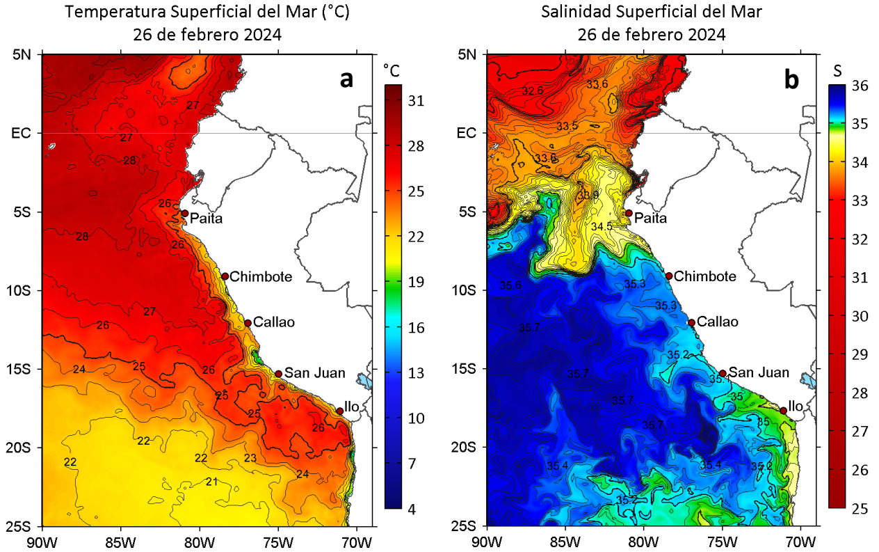
Figura 2. a) Temperatura superficial del mar ( ^{\circ}\text{C} ) y b) Salinidad superficial del mar para el 26 de febrero de 2024. Datos: OSTIA-UKMO-L4-GLOB-v2.0 (UK Met Office, 2012; Donlon et al, 2012) y del GLOBAL_ANALYSISFORECAST_PHY_001_024 (Lellouche, J. M. et al, 2013), respectivamente.
