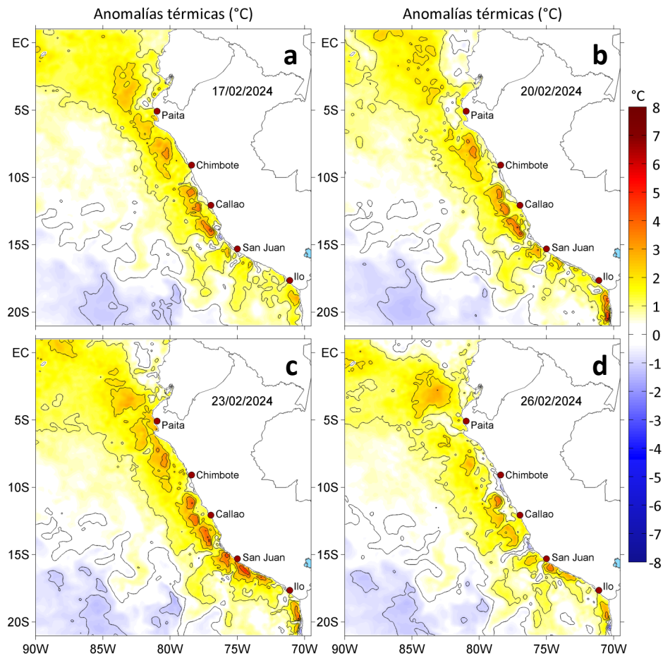
Figura 3. Anomalías de la temperatura superficial del mar ( ^{\circ}\text{C} ) para el a) 17, b) 20, c) 23 y d) 26 de febrero de 2024. Las anomalías se calcularon respecto de la climatología para el periodo 1991-2020. Datos: OSTIA-UKMO-L4-GLOB-v2.0 (UK Met Office, 2012; Donlon et al, 2012).
