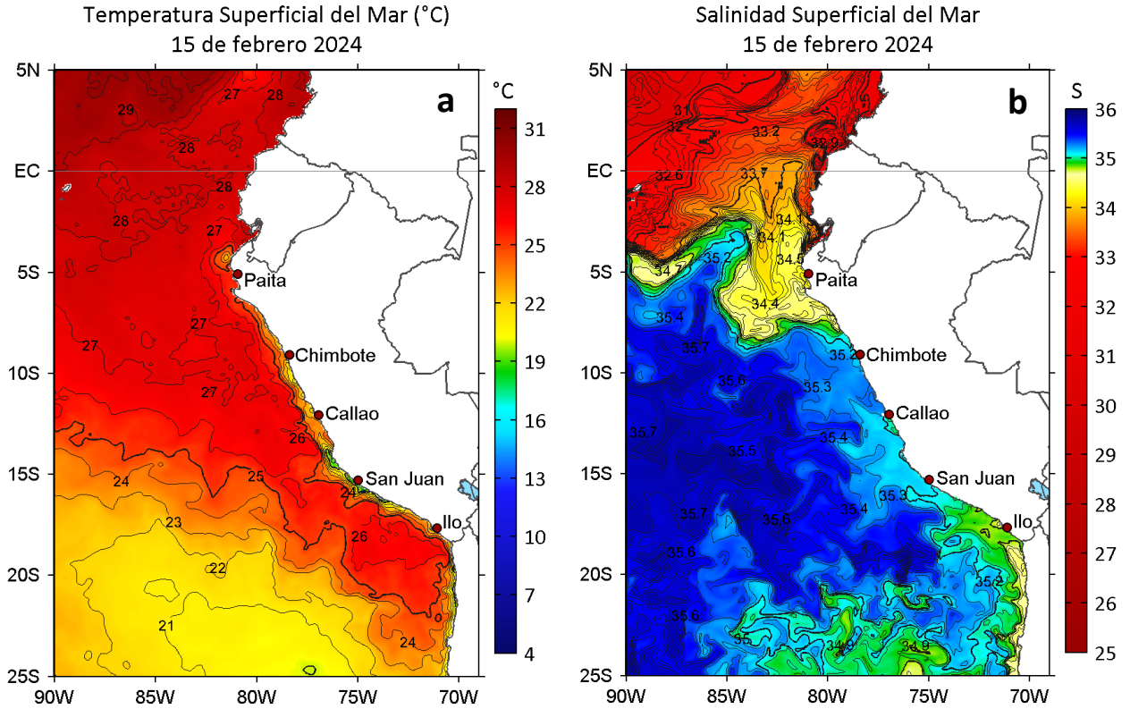
Figura 2. a) Temperatura superficial del mar ( ^{\circ}\text{C} ) y b) Salinidad superficial del mar para el 15 de febrero de 2024. Datos: OSTIA-UKMO-L4-GLOB-v2.0 (UK Met Office, 2012; Donlon et al, 2012) y del GLOBAL_ANALYSISFORECAST_PHY_001_024 (Lellouche, J. M. et al, 2013), respectivamente.
