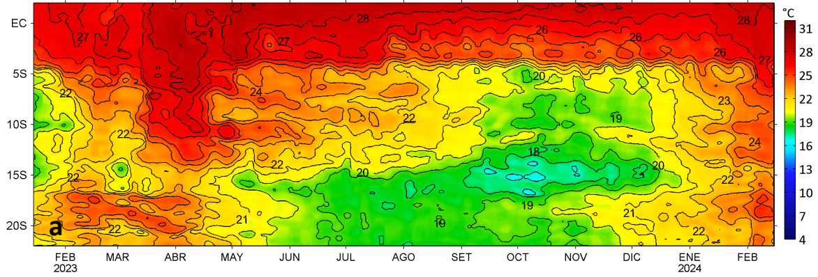
Anomalías de la Temperatura Superficial del mar (°C), franja costera de 60 mn 15 de enero 2023 - 15 de febrero 2024
