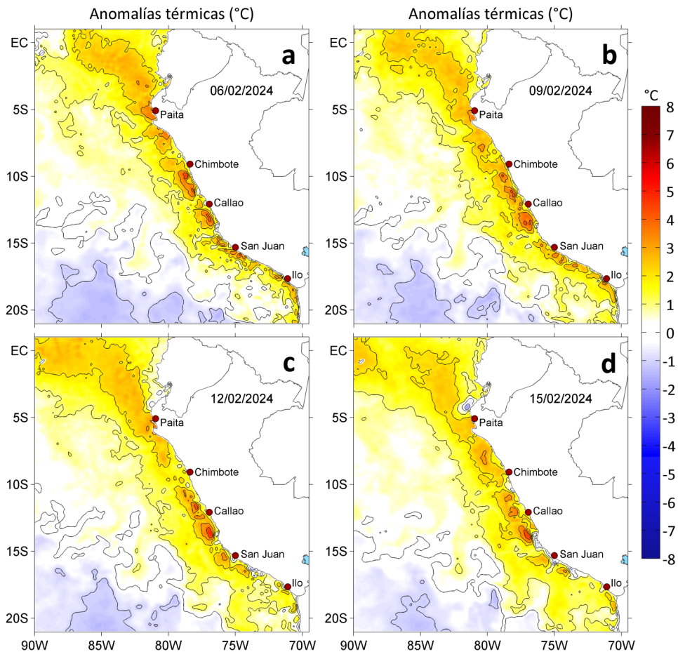
Figura 3. Anomalías de la temperatura superficial del mar ( ^{\circ}\text{C} ) para el a) 06, b) 09, c) 12 y d) 15 de febrero de 2024. Las anomalías se calcularon respecto de la climatología para el periodo 1991-2020. Datos: OSTIA-UKMO-L4-GLOB-v2.0 (UK Met Office, 2012; Donlon et al, 2012).
