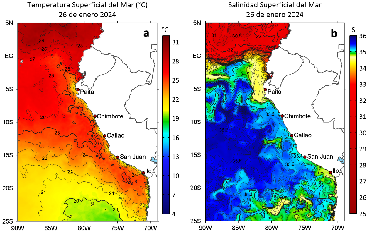
Figura 2. a) Temperatura superficial del mar ( ^{\circ}\text{C} ) y b) Salinidad superficial del mar para el 26 de enero de 2024. Datos: OSTIA-UKMO-L4-GLOB-v2.0 (UK Met Office, 2012; Donlon et al, 2012) y del GLOBAL_ANALYSISFORECAST_PHY_001_024 (Lellouche, J. M. et al, 2013), respectivamente.
