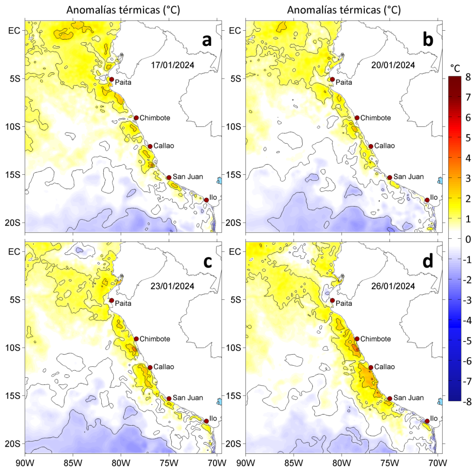
Figura 3. Anomalías de la temperatura superficial del mar ( ^{\circ}\text{C} ) para el a) 17, b) 20, c) 23 y d) 26 de enero de 2024. Las anomalías se calcularon respecto de la climatología para el periodo 1991-2020. Datos: OSTIA-UKMO-L4-GLOB-v2.0 (UK Met Office, 2012; Donlon et al, 2012).
