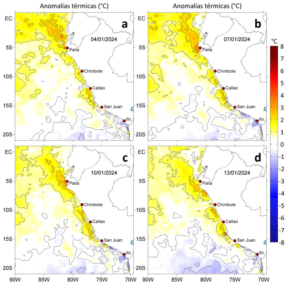
Figura 3. Anomalías de la temperatura superficial del mar ( ^{\circ}\text{C} ) para el a) 04, b) 07, c) 10 y d) 13 de enero de 2024. Las anomalías se calcularon respecto de la climatología para el periodo 1991-2020. Datos: OSTIA-UKMO-L4-GLOB-v2.0 (UK Met Office, 2012; Donlon et al, 2012).
