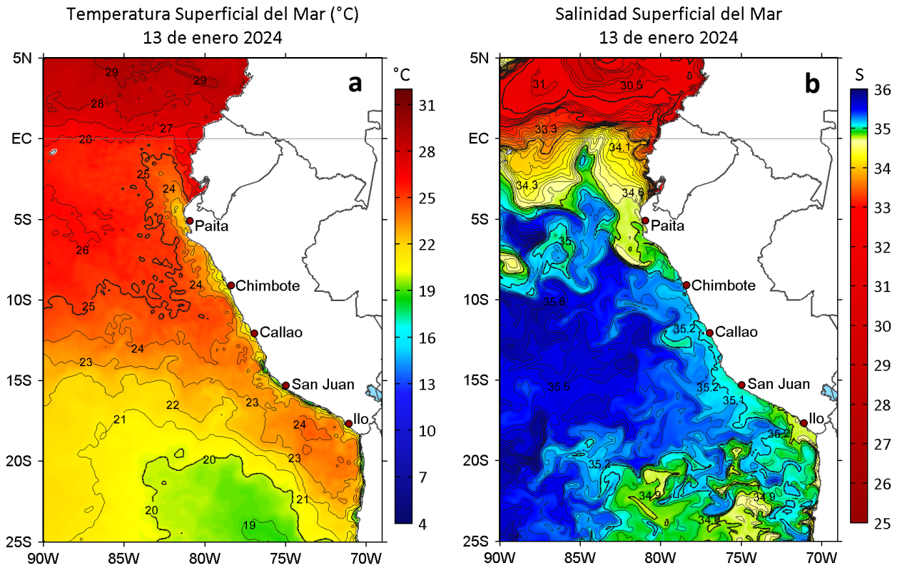
Figura 2. a) Temperatura superficial del mar ( ^{\circ}\text{C} ) y b) Salinidad superficial del mar para el 13 de enero de 2024. Datos: OSTIA-UKMO-L4-GLOB-v2.0 (UK Met Office, 2012; Donlon et al, 2012) y del GLOBAL_ANALYSISFORECAST_PHY_001_024 (Lellouche, J. M. et al, 2013), respectivamente.
