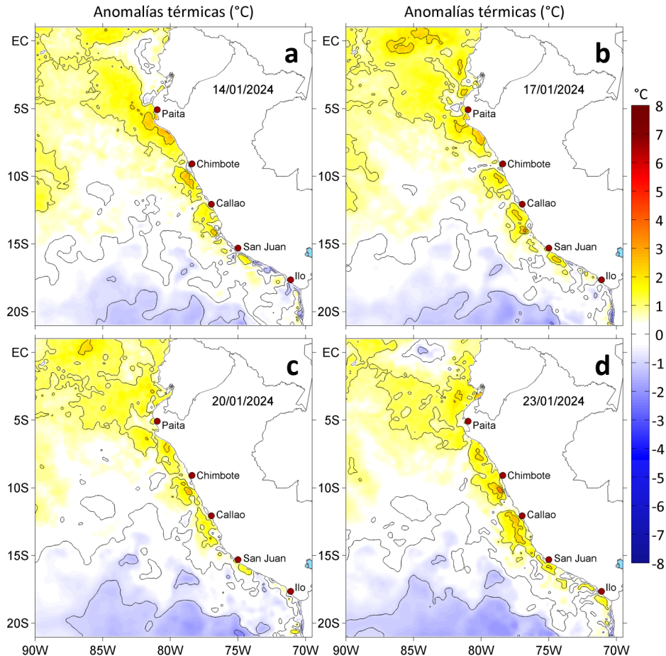
Figura 3. Anomalías de la temperatura superficial del mar (°C) para el a) 14, b) 17, c) 20 y d) 23 de enero de 2024. Las anomalías se calcularon respecto de la climatología para el periodo 1991-2020. Datos: OSTIA-UKMO-L4-GLOB-v2.0 (UK Met Office, 2012; Donlon et al, 2012).
