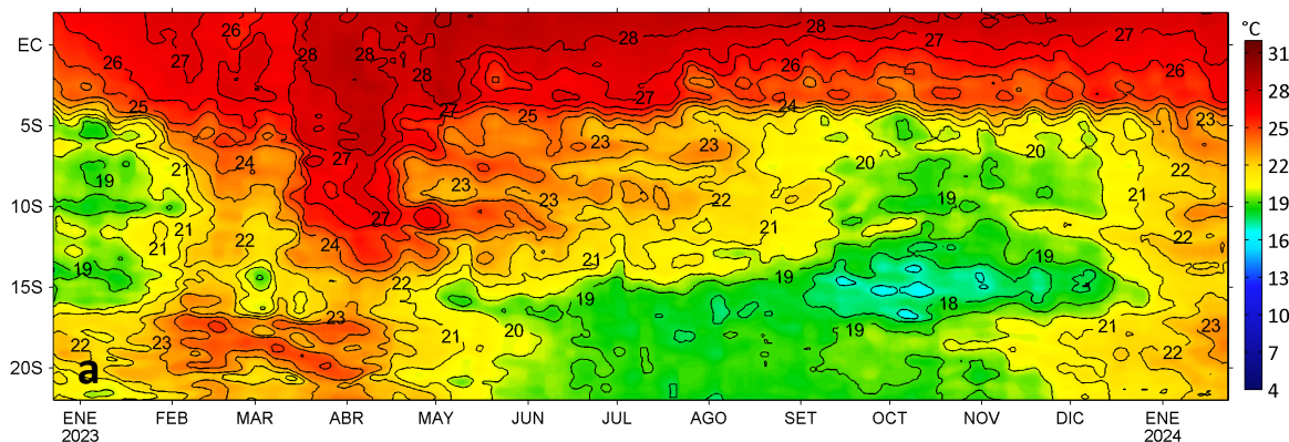
Anomalías de la Temperatura Superficial del mar (°C), franja costera de 60 mn 23 de diciembre 2022 - 23 de enero 2024
