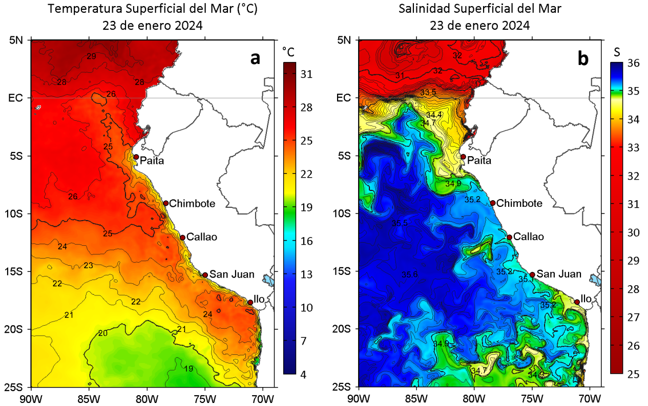
Figura 2. a) Temperatura superficial del mar (°C) y b) Salinidad superficial del mar para el 23 de enero de 2024. Datos: OSTIA-UKMO-L4-GLOB-v2.0 (UK Met Office, 2012; Donlon et al, 2012) y del GLOBAL_ANALYSISFORECAST_PHY_001_024 (Lellouche, J. M. et al, 2013), respectivamente.
