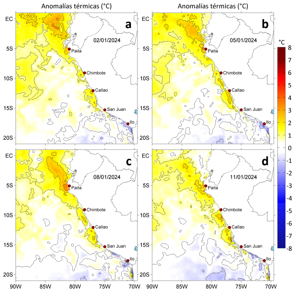
Figura 3. Anomalías de la temperatura superficial del mar ( ^{\circ}\text{C} ) para el a) 02, b) 05, c) 08 y d) 11 de enero de 2024. Las anomalías se calcularon respecto de la climatología para el periodo 1991-2020. Datos: OSTIA-UKMO-L4-GLOB-v2.0 (UK Met Office, 2012; Donlon et al, 2012).
