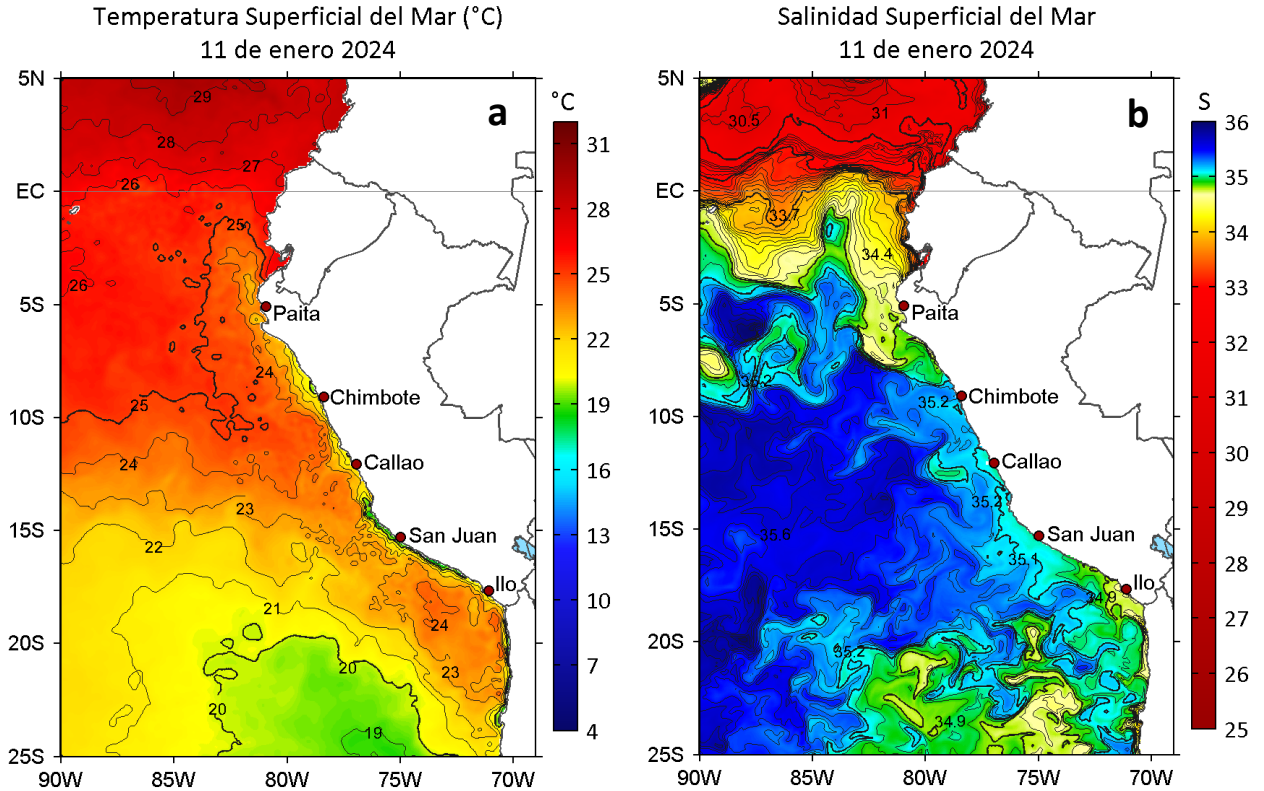
Figura 2. a) Temperatura superficial del mar ( ^{\circ}\text{C} ) y b) Salinidad superficial del mar para el 11 de enero de 2024. Datos: OSTIA-UKMO-L4-GLOB-v2.0 (UK Met Office, 2012; Donlon et al, 2012) y del GLOBAL_ANALYSISFORECAST_PHY_001_024 (Lellouche, J. M. et al, 2013), respectivamente.
