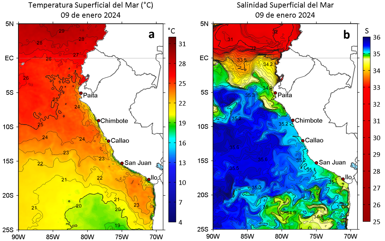
Figura 2. a) Temperatura superficial del mar (°C) y b) Salinidad superficial del mar para el 09 de enero de 2024. Datos: OSTIA-UKMO-L4-GLOB-v2.0 (UK Met Office, 2012; Donlon et al, 2012) y del GLOBAL_ANALYSISFORECAST_PHY_001_024 (Lellouche, J. M. et al, 2013), respectivamente.
