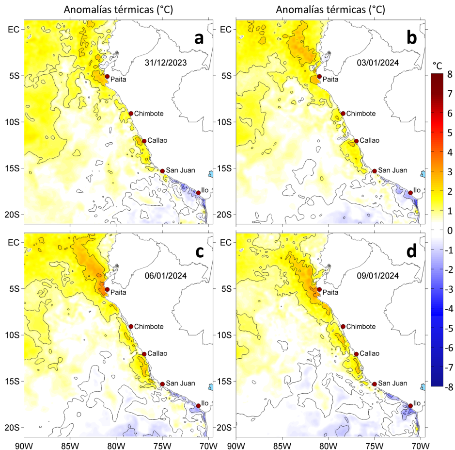
Figura 3. Anomalías de la temperatura superficial del mar (°C) para el a) 31 de diciembre de 2023, b) 03, c) 06 y d) 09 de enero de 2024. Las anomalías se calcularon respecto de la climatología para el periodo 1991-2020. Datos: OSTIA-UKMO-L4-GLOB-v2.0 (UK Met Office, 2012; Donlon et al, 2012).
