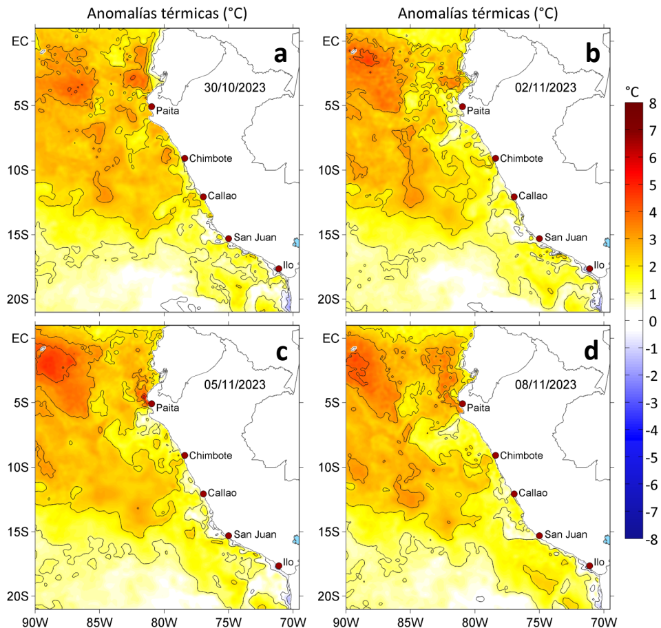
Figura 3. Anomalías de la temperatura superficial del mar ( ^{\circ}\text{C} ) para el a) 30 de octubre, b) 02, c) 05 y d) 08 de noviembre de 2023. Las anomalías se calcularon respecto de la climatología para el periodo 1991-2020. Datos: OSTIA-UKMO-L4-GLOB-v2.0 (UK Met Office, 2012; Donlon et al, 2012).
