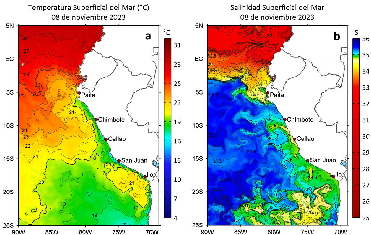
Figura 2. a) Temperatura superficial del mar ( ^{\circ}\text{C} ) y b) Salinidad superficial del mar para el 08 de noviembre de 2023. Datos: OSTIA-UKMO-L4-GLOB-v2.0 (UK Met Office, 2012; Donlon et al, 2012) y del GLOBAL_ANALYSISFORECAST_PHY_001_024 (Lellouche, J. M. et al, 2013), respectivamente.
