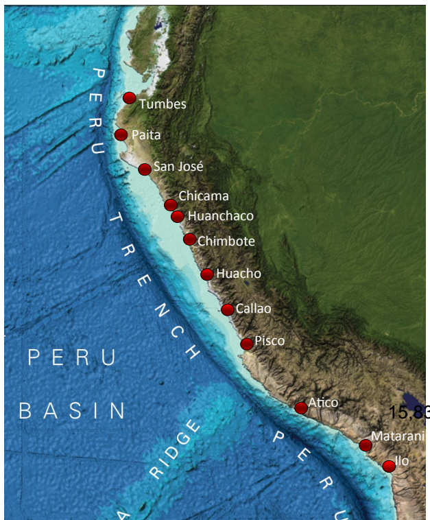
Figura 1. Localización de las estaciones oceanográficas del IMARPE (en círculos de color rojo) en el litoral peruano. El mapa fue adaptado de GEBCO (2014).
