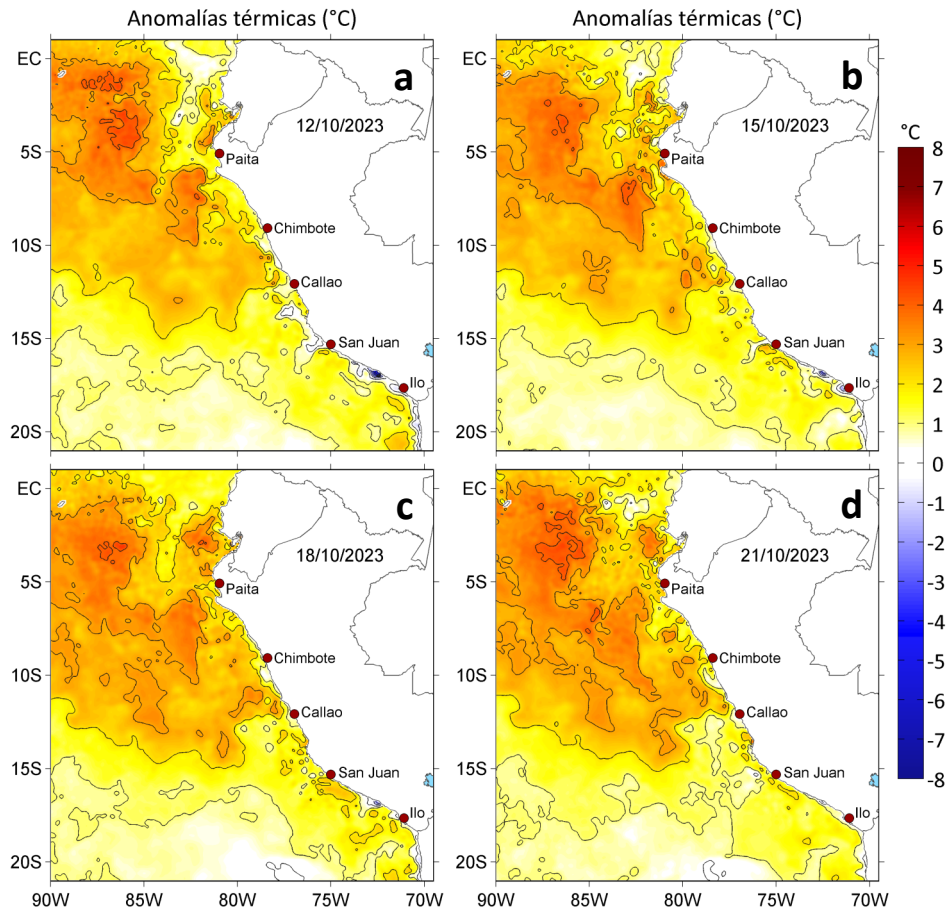
Figura 3. Anomalías de la temperatura superficial del mar ( ^{\circ}\text{C} ) para el a) 12, b) 15, c) 18 y d) 21 de octubre de 2023. Las anomalías se calcularon respecto de la climatología para el periodo 1991-2020. Datos: OSTIA-UKMO-L4-GLOB-v2.0 (UK Met Office, 2012; Donlon et al, 2012).
