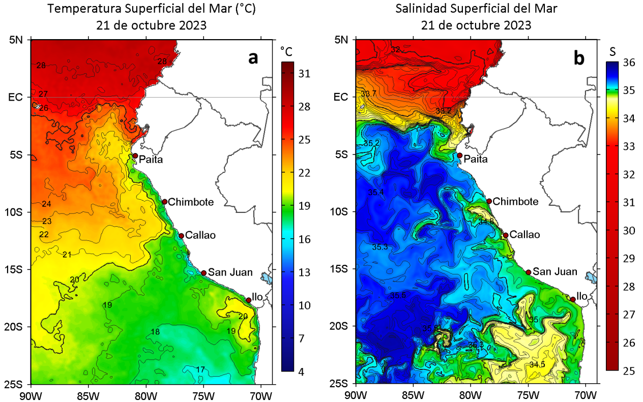
Figura 2. a) Temperatura superficial del mar ( ^{\circ}\text{C} ) y b) Salinidad superficial del mar para el 21 de octubre de 2023. Datos: OSTIA-UKMO-L4-GLOB-v2.0 (UK Met Office, 2012; Donlon et al, 2012) y del GLOBAL_ANALYSISFORECAST_PHY_001_024 (Lellouche, J. M. et al, 2013), respectivamente.
