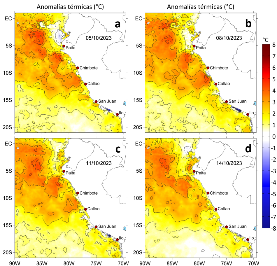
Figura 3. Anomalías de la temperatura superficial del mar ( ^{\circ}\text{C} ) para el a) 05, b) 08, c) 11 y d) 14 de octubre de 2023. Las anomalías se calcularon respecto de la climatología para el periodo 1991-2020. Datos: OSTIA-UKMO-L4-GLOB-v2.0 (UK Met Office, 2012; Donlon et al, 2012).
