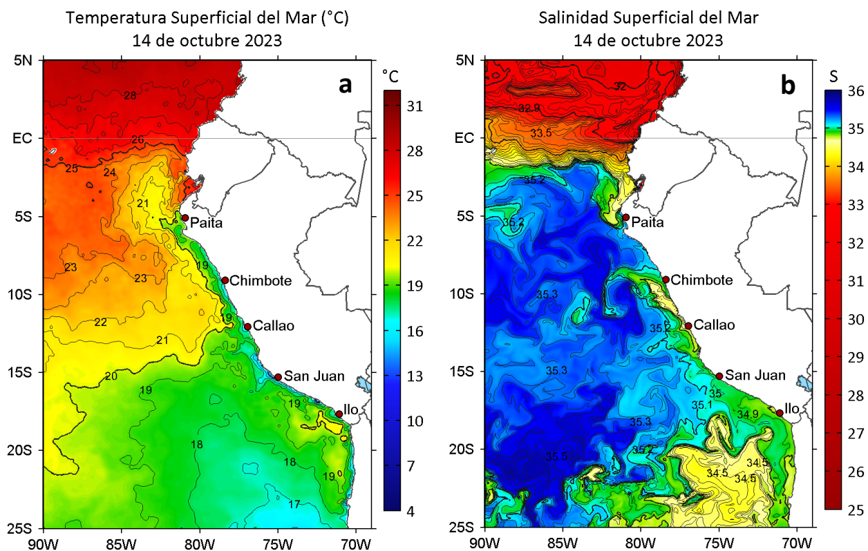
Figura 2. a) Temperatura superficial del mar ( ^{\circ}\text{C} ) y b) Salinidad superficial del mar para el 14 de octubre de 2023. Datos: OSTIA-UKMO-L4-GLOB-v2.0 (UK Met Office, 2012; Donlon et al, 2012) y del GLOBAL_ANALYSISFORECAST_PHY_001_024 (Lellouche, J. M. et al, 2013), respectivamente.
