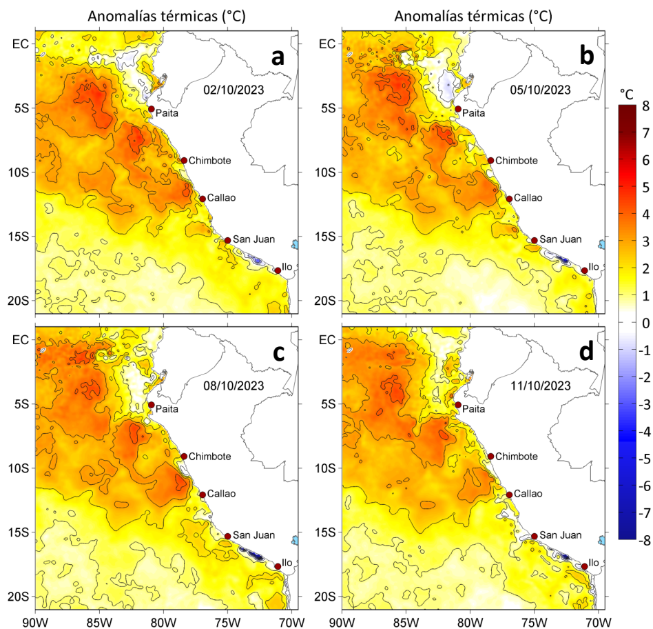
Figura 3. Anomalías de la temperatura superficial del mar ( ^{\circ}\text{C} ) para el a) 02, b) 05, c) 08 y d) 11 de octubre de 2023. Las anomalías se calcularon respecto de la climatología para el periodo 1991-2020. Datos: OSTIA-UKMO-L4-GLOB-v2.0 (UK Met Office, 2012; Donlon et al, 2012).
