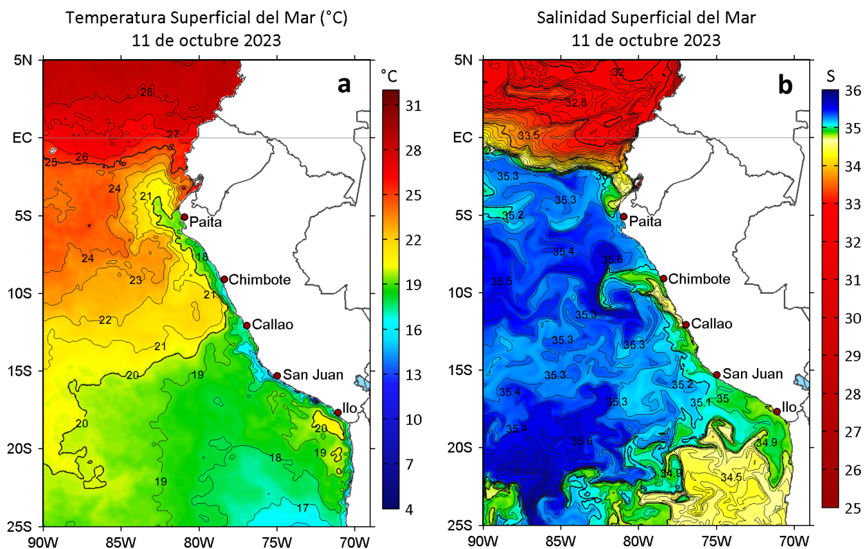
Figura 2. a) Temperatura superficial del mar ( ^{\circ}\text{C} ) y b) Salinidad superficial del mar para el 11 de octubre de 2023. Datos: OSTIA-UKMO-L4-GLOB-v2.0 (UK Met Office, 2012; Donlon et al, 2012) y del GLOBAL_ANALYSISFORECAST_PHY_001_024 (Lellouche, J. M. et al, 2013), respectivamente.
