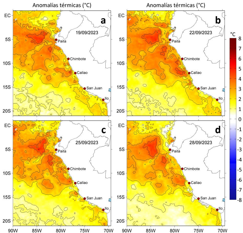
Figura 3. Anomalías de la temperatura superficial del mar (°C) para el a) 19, b) 22, c) 25 y d) 28 de setiembre de 2023. Las anomalías se calcularon respecto de la climatología para el periodo 1991-2020. Datos: OSTIA-UKMO-L4-GLOB-v2.0 (UK Met Office, 2012; Donlon et al, 2012).
