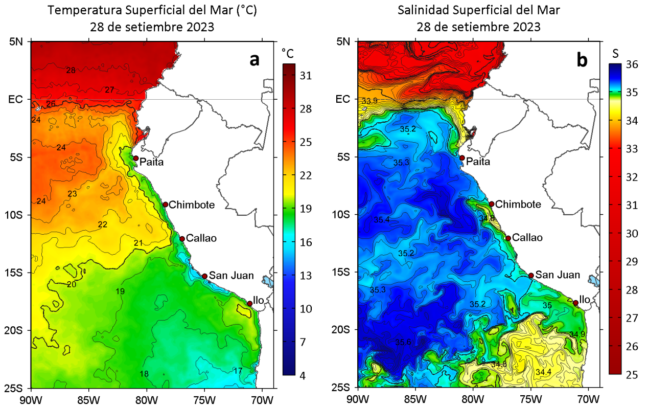
Figura 2. a) Temperatura superficial del mar (°C) y b) Salinidad superficial del mar para el 28 de setiembre de 2023. Datos: OSTIA-UKMO-L4-GLOB-v2.0 (UK Met Office, 2012; Donlon et al, 2012) y del GLOBAL_ANALYSISFORECAST_PHY_001_024 (Lellouche, J. M. et al, 2013), respectivamente.
