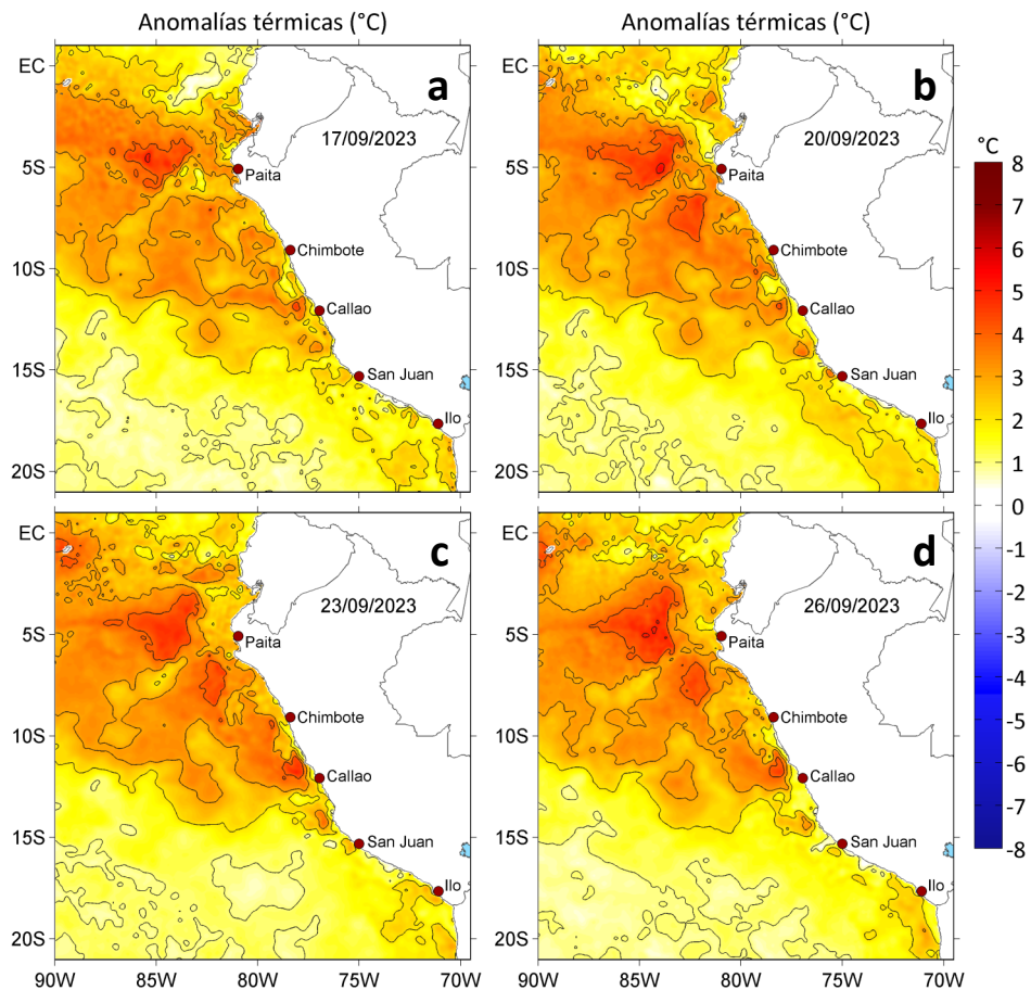
Figura 3. Anomalías de la temperatura superficial del mar ( ^{\circ}\text{C} ) para el a) 17, b) 20, c) 23 y d) 26 de setiembre de 2023. Las anomalías se calcularon respecto de la climatología para el periodo 1991-2020. Datos: OSTIA-UKMO-L4-GLOB-v2.0 (UK Met Office, 2012; Donlon et al, 2012).
