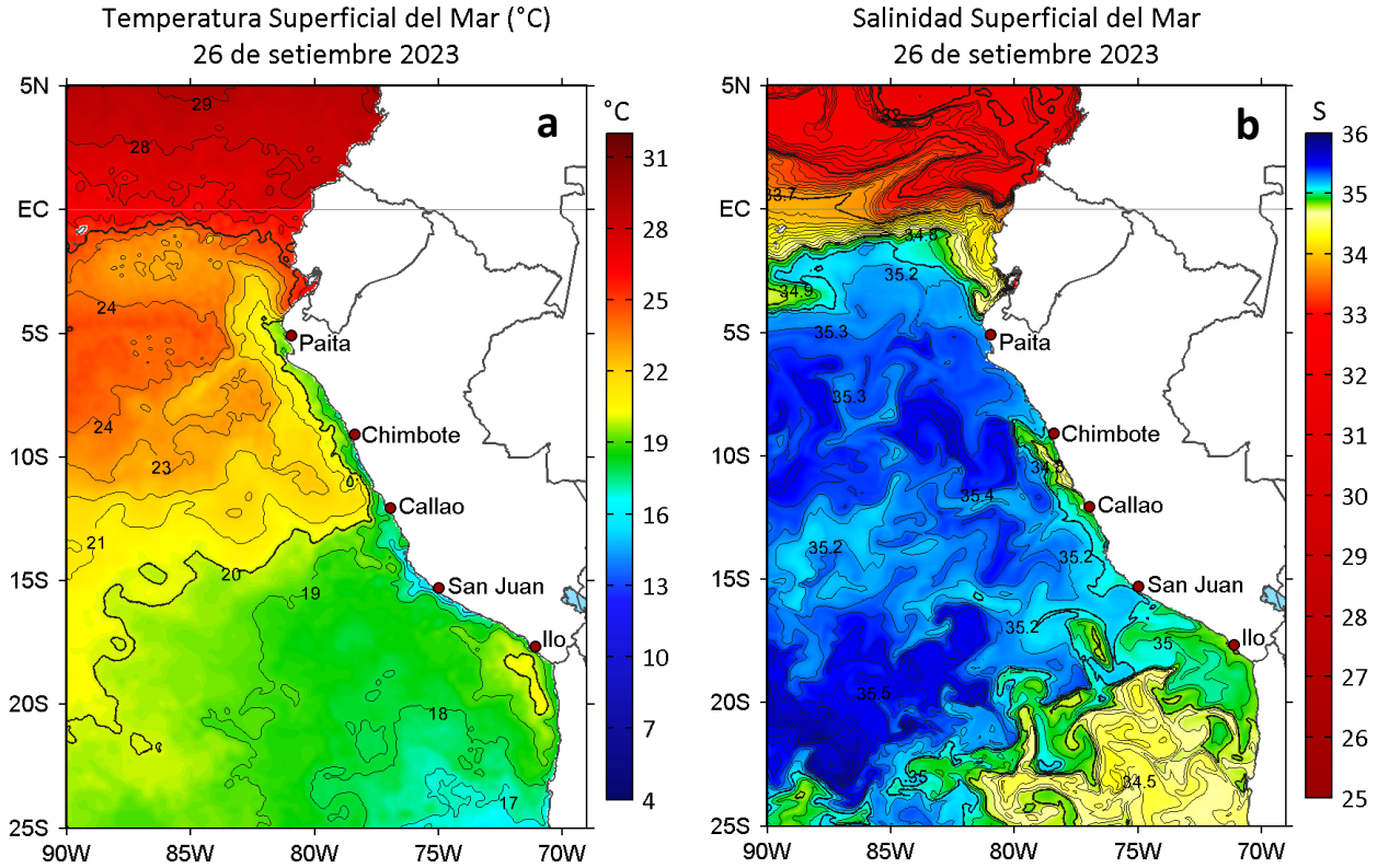
Figura 2. a) Temperatura superficial del mar ( ^{\circ}\text{C} ) y b) Salinidad superficial del mar para el 26 de setiembre de 2023. Datos: OSTIA-UKMO-L4-GLOB-v2.0 (UK Met Office, 2012; Donlon et al, 2012) y del GLOBAL_ANALYSISFORECAST_PHY_001_024 (Lellouche, J. M. et al, 2013), respectivamente.
