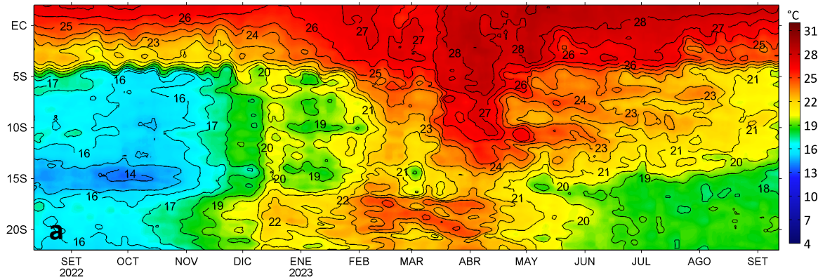
Anomalías de la Temperatura Superficial del mar (°C), franja costera de 60 mn 12 de agosto 2022 - 12 de setiembre 2023
