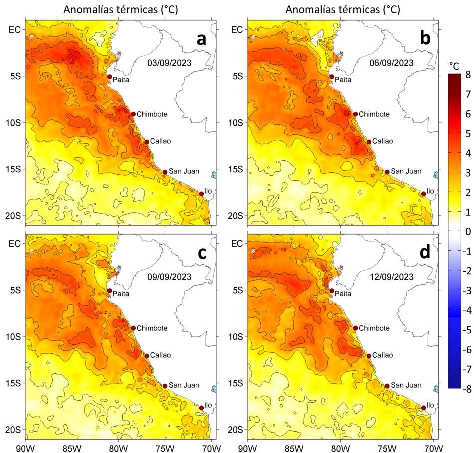
Figura 3. Anomalías de la temperatura superficial del mar ( ^{\circ}\text{C} ) para el a) 03, b) 06, c) 09 y d) 12 de setiembre de 2023. Las anomalías se calcularon respecto de la climatología para el periodo 1991-2020. Datos: OSTIA-UKMO-L4-GLOB-v2.0 (UK Met Office, 2012; Donlon et al, 2012).
