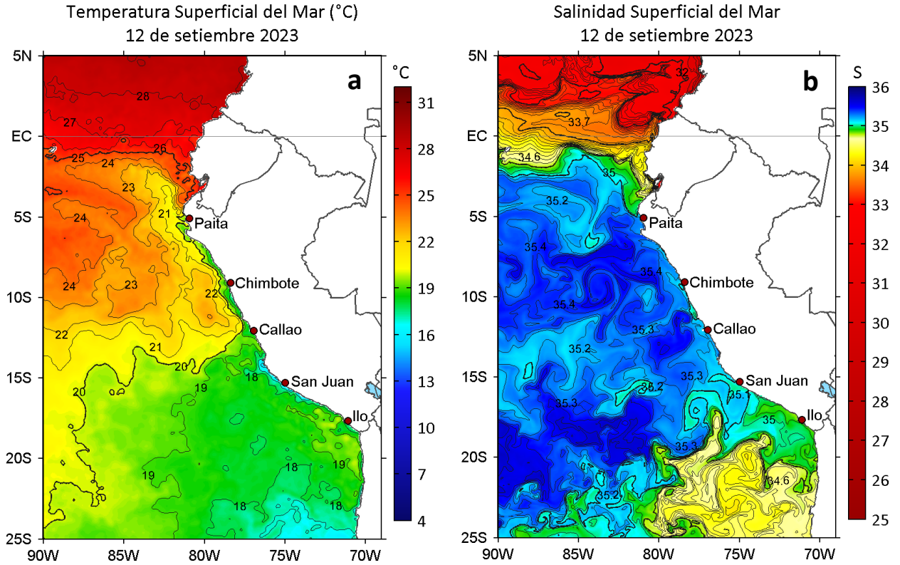
Figura 2. a) Temperatura superficial del mar ( ^{\circ}\text{C} ) y b) Salinidad superficial del mar para el 12 de setiembre de 2023. Datos: OSTIA-UKMO-L4-GLOB-v2.0 (UK Met Office, 2012; Donlon et al, 2012) y del GLOBAL_ANALYSISFORECAST_PHY_001_024 (Lellouche, J. M. et al, 2013), respectivamente.
