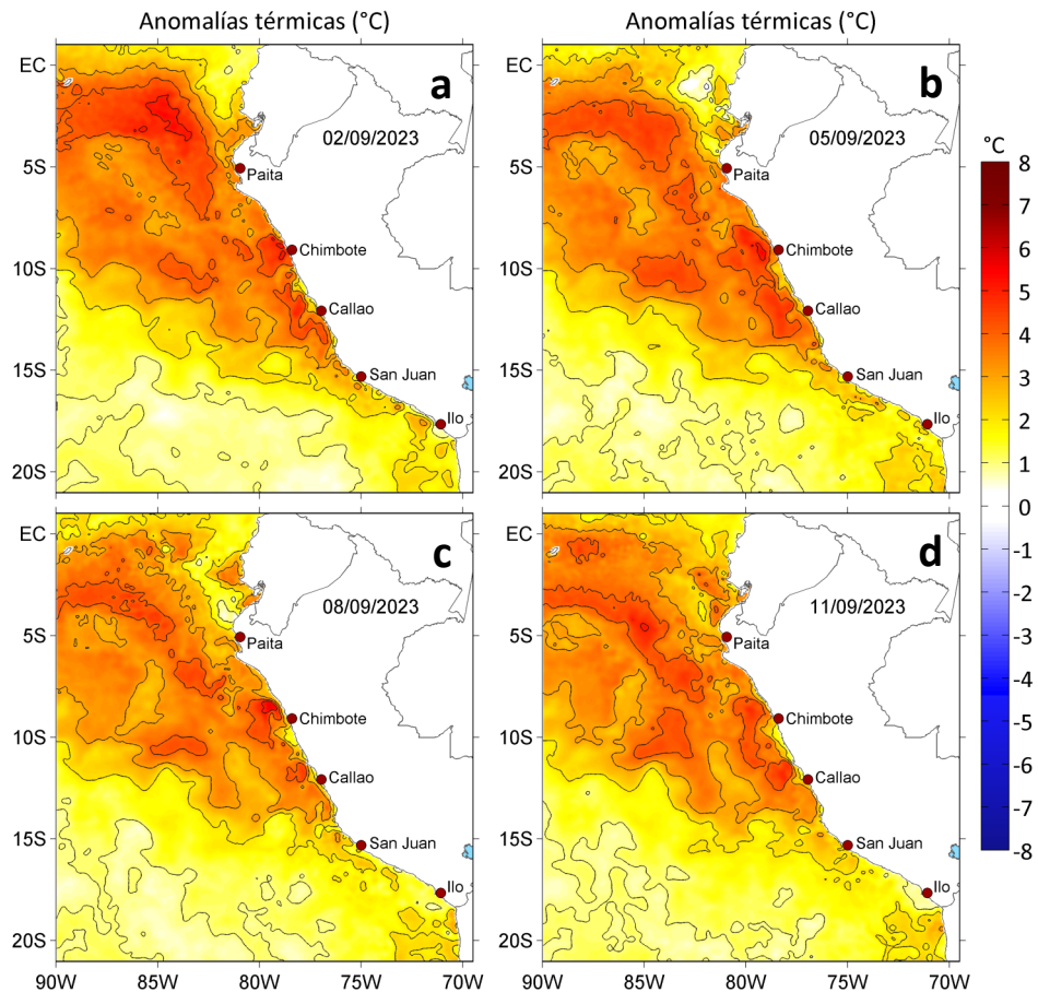
Figura 3. Anomalías de la temperatura superficial del mar ( ^{\circ}\text{C} ) para el a) 02, b) 05, c) 08 y d) 11 de setiembre de 2023. Las anomalías se calcularon respecto de la climatología para el periodo 1991-2020. Datos: OSTIA-UKMO-L4-GLOB-v2.0 (UK Met Office, 2012; Donlon et al, 2012).
