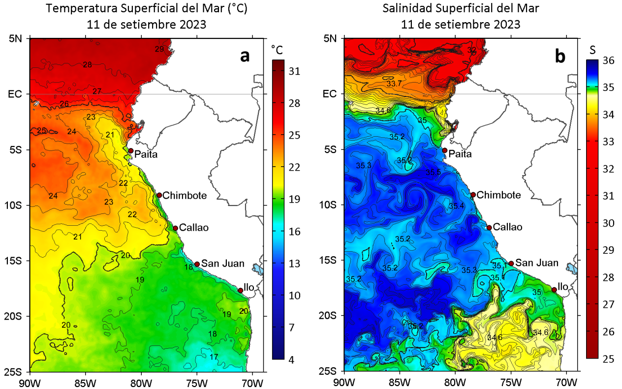
Figura 2. a) Temperatura superficial del mar ( ^{\circ}\text{C} ) y b) Salinidad superficial del mar para el 11 de setiembre de 2023. Datos: OSTIA-UKMO-L4-GLOB-v2.0 (UK Met Office, 2012; Donlon et al, 2012) y del GLOBAL_ANALYSISFORECAST_PHY_001_024 (Lellouche, J. M. et al, 2013), respectivamente.
