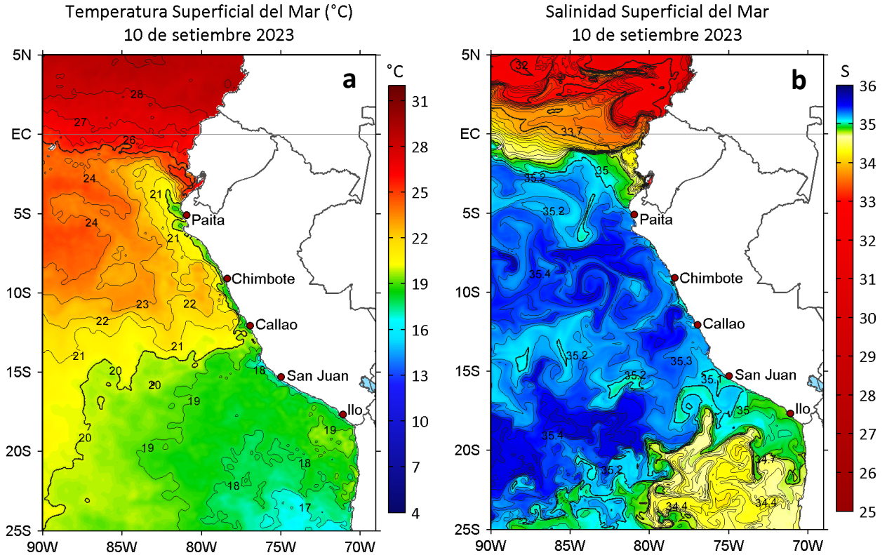
Figura 2. a) Temperatura superficial del mar ( ^{\circ}\text{C} ) y b) Salinidad superficial del mar para el 10 de setiembre de 2023. Datos: OSTIA-UKMO-L4-GLOB-v2.0 (UK Met Office, 2012; Donlon et al, 2012) y del GLOBAL_ANALYSISFORECAST_PHY_001_024 (Lellouche, J. M. et al, 2013), respectivamente.
