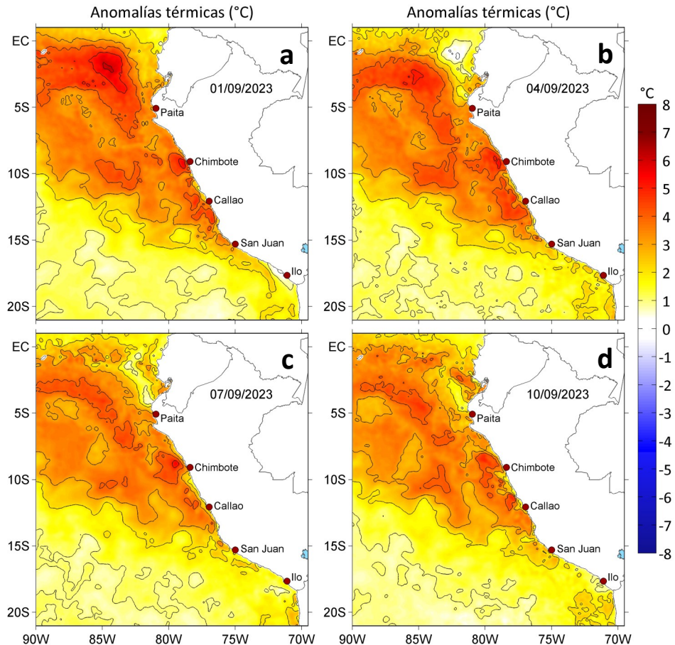
Figura 3. Anomalías de la temperatura superficial del mar ( ^{\circ}\text{C} ) para el a) 01, b) 04, c) 07 y d) 10 de setiembre de 2023. Las anomalías se calcularon respecto de la climatología para el periodo 1991-2020. Datos: OSTIA-UKMO-L4-GLOB-v2.0 (UK Met Office, 2012; Donlon et al, 2012).
