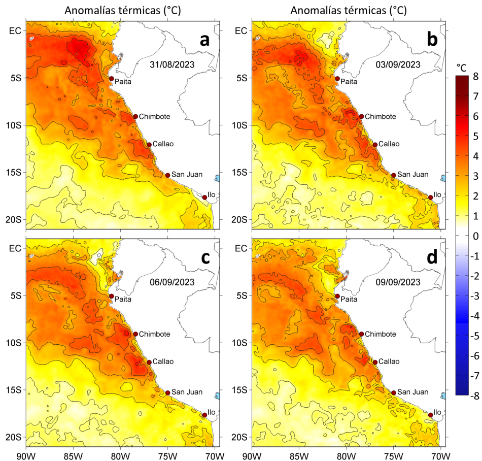
Figura 3. Anomalías de la temperatura superficial del mar ( ^{\circ}\text{C} ) para el a) 31 de agosto, b) 03, c) 06 y d) 09 de setiembre de 2023. Las anomalías se calcularon respecto de la climatología para el periodo 1991-2020. Datos: OSTIA-UKMO-L4-GLOB-v2.0 (UK Met Office, 2012; Donlon et al, 2012).
