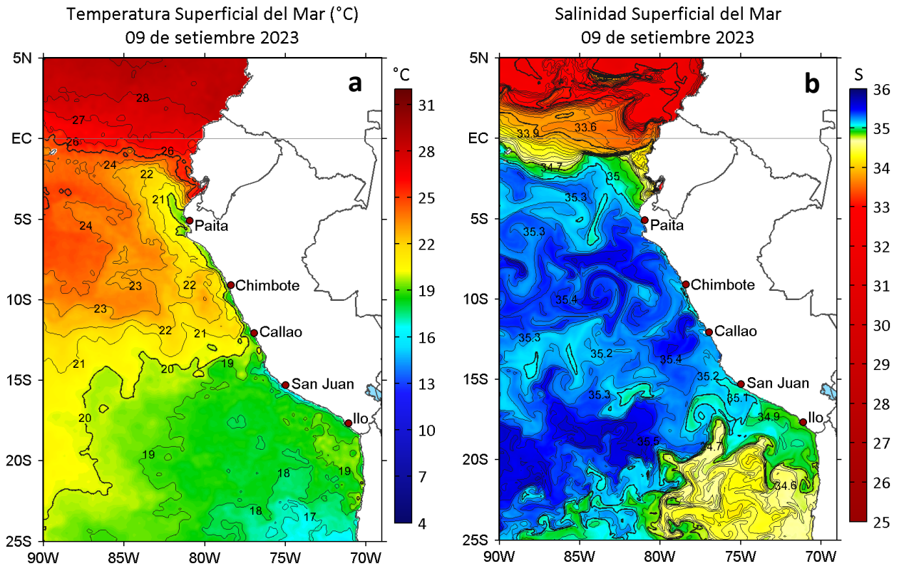
Figura 2. a) Temperatura superficial del mar ( ^{\circ}\text{C} ) y b) Salinidad superficial del mar para el 09 de setiembre de 2023. Datos: OSTIA-UKMO-L4-GLOB-v2.0 (UK Met Office, 2012; Donlon et al, 2012) y del GLOBAL_ANALYSISFORECAST_PHY_001_024 (Lellouche, J. M. et al, 2013), respectivamente.
