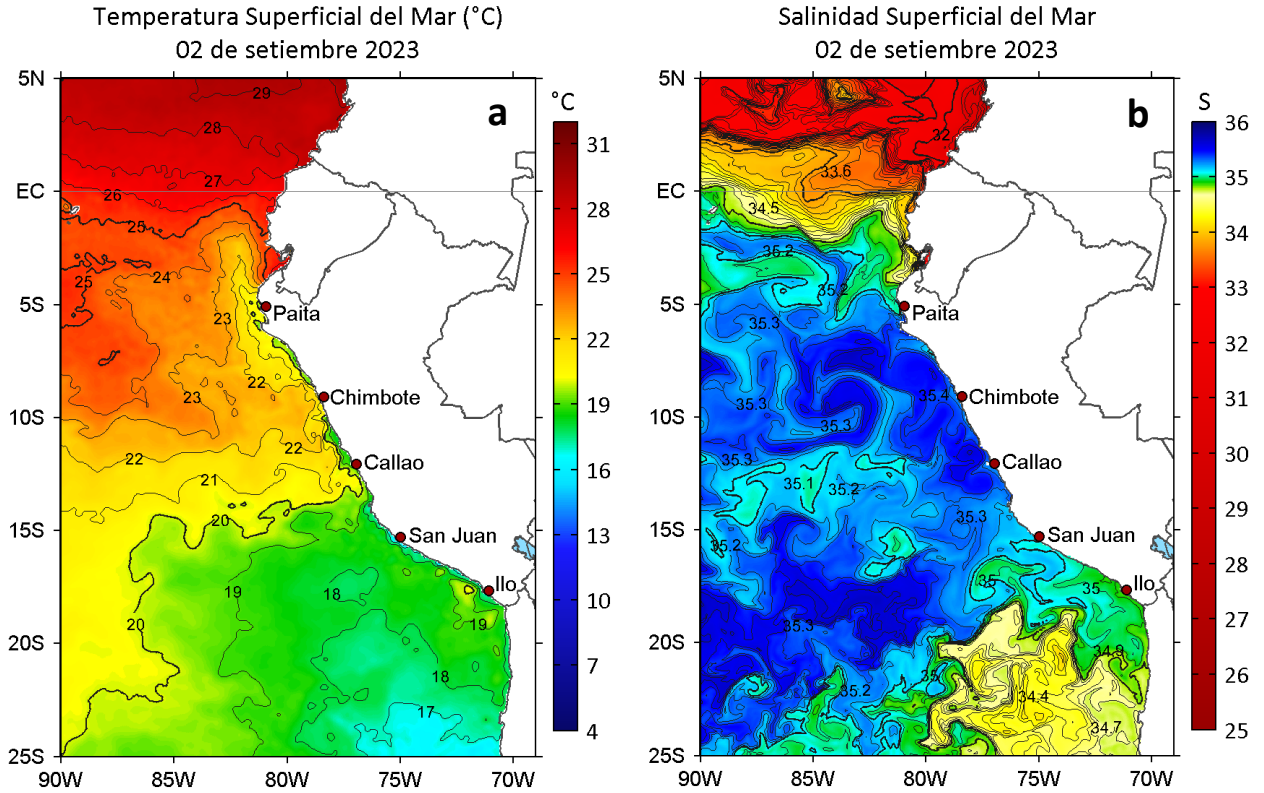
Figura 2. a) Temperatura superficial del mar ( ^{\circ}\text{C} ) y b) Salinidad superficial del mar para el 02 de setiembre de 2023. Datos: OSTIA -UKMO-L4-GLOB-v2.0 (UK Met Office, 2012; Donlon et al, 2012) y del GLOBAL_ANALYSISFORECAST_PHY_001_024 (Lellouche, J. M. et al, 2013), respectivamente.
