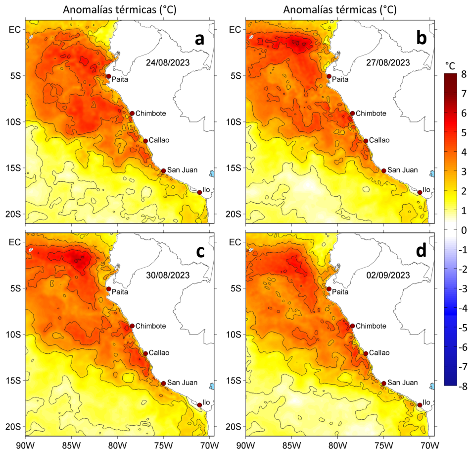
Figura 3. Anomalías de la temperatura superficial del mar ( ^{\circ}\text{C} ) para el a) 24, b) 27 y c) 30 de agosto, así como para el d) 02 de setiembre de 2023. Las anomalías se calcularon respecto de la climatología para el periodo 1991-2020. Datos: OSTIA-UKMO-L4-GLOB-v2.0 (UK Met Office, 2012; Donlon et al, 2012).
