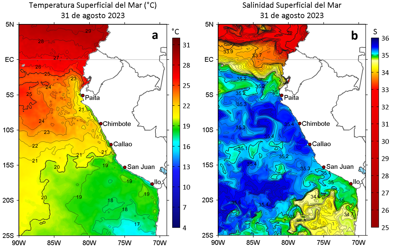
Figura 2. a) Temperatura superficial del mar ( ^{\circ}\text{C} ) y b) Salinidad superficial del mar para el 31 de agosto de 2023. Datos: OSTIA-UKMO-L4-GLOB-v2.0 (UK Met Office, 2012; Donlon et al, 2012) y del GLOBAL_ANALYSISFORECAST_PHY_001_024 (Lellouche, J. M. et al, 2013), respectivamente.
