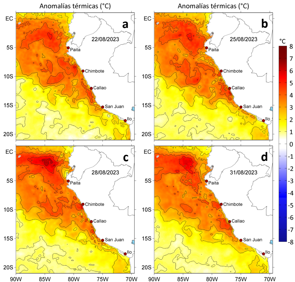
Figura 3. Anomalías de la temperatura superficial del mar ( ^{\circ}\text{C} ) para el a) 22, b) 25, c) 28 y d) 31 de agosto de 2023. Las anomalías se calcularon respecto de la climatología para el periodo 1991-2020. Datos: OSTIA-UKMO-L4-GLOB-v2.0 (UK Met Office, 2012; Donlon et al, 2012).
