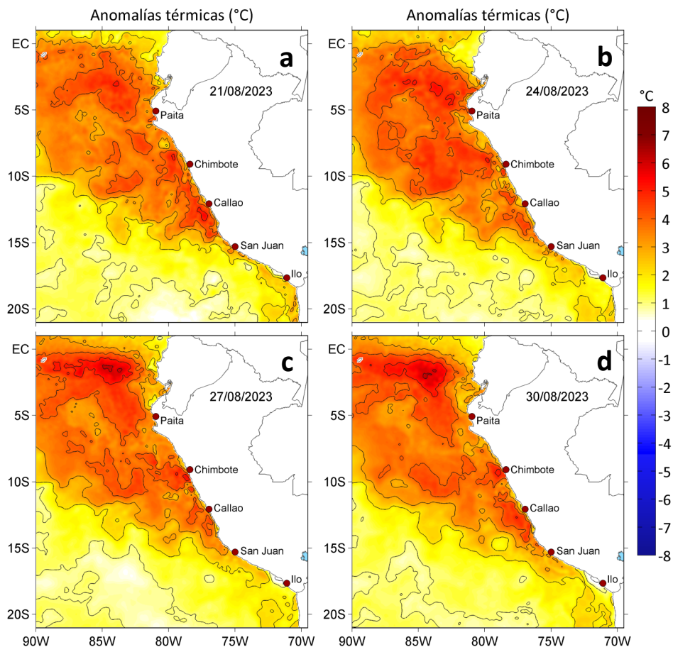
Figura 3. Anomalías de la temperatura superficial del mar ( ^{\circ}\text{C} ) para el a) 21, b) 24, c) 27 y d) 30 de agosto de 2023. Las anomalías se calcularon respecto de la climatología para el periodo 1991-2020. Datos: OSTIA-UKMO-L4-GLOB-v2.0 (UK Met Office, 2012; Donlon et al, 2012).
