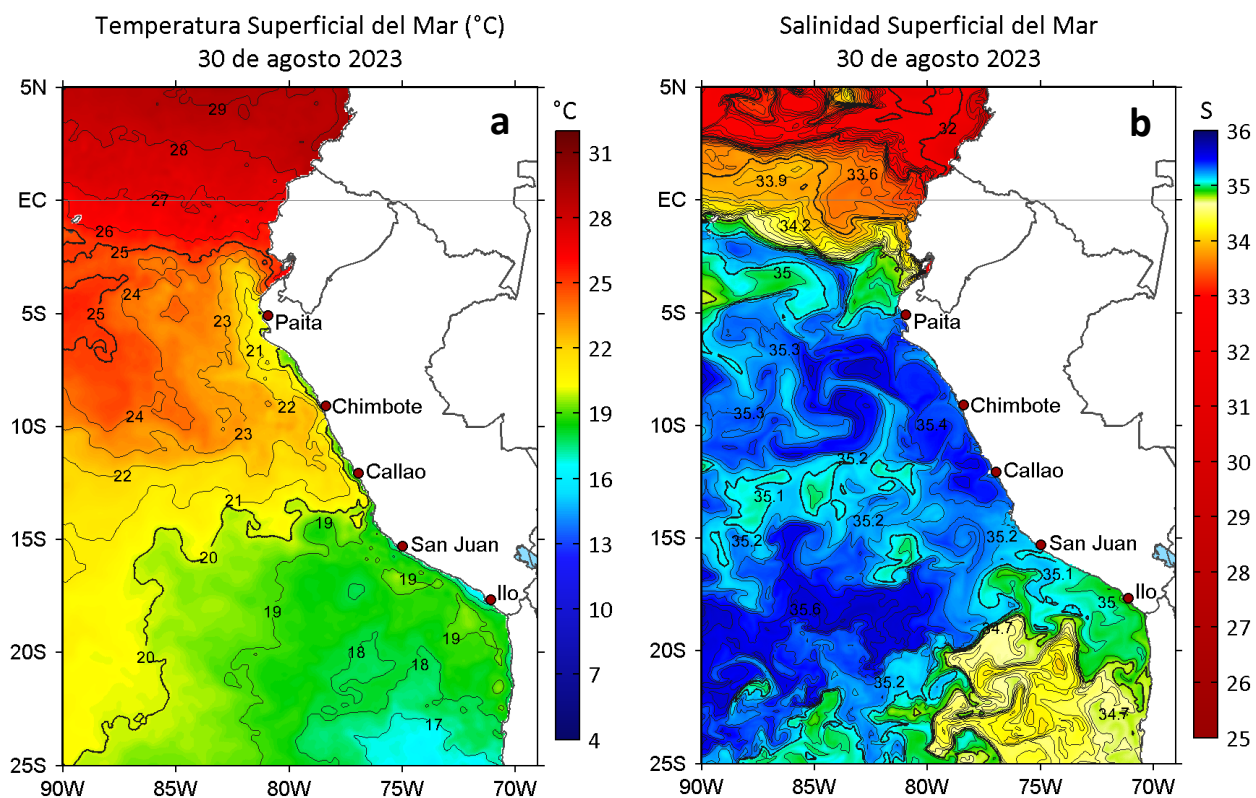
Figura 2. a) Temperatura superficial del mar ( ^{\circ}\text{C} ) y b) Salinidad superficial del mar para el 30 de agosto de 2023. Datos: OSTIA-UKMO-L4-GLOB-v2.0 (UK Met Office, 2012; Donlon et al, 2012) y del GLOBAL_ANALYSISFORECAST_PHY_001_024 (Lellouche, J. M. et al, 2013), respectivamente.
