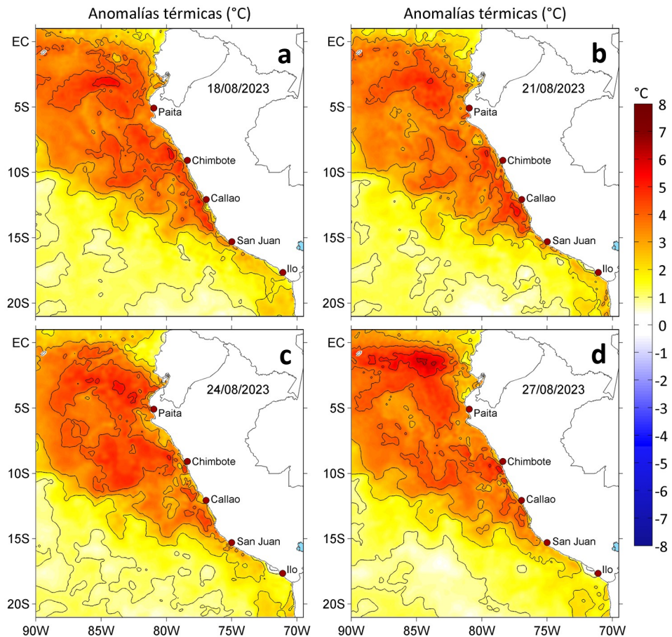
Figura 3. Anomalías de la temperatura superficial del mar ( ^{\circ}\text{C} ) para el a) 18, b) 21, c) 24 y d) 27 de agosto de 2023. Las anomalías se calcularon respecto de la climatología para el periodo 1991-2020. Datos: OSTIA-UKMO-L4-GLOB-v2.0 (UK Met Office, 2012; Donlon et al, 2012).
