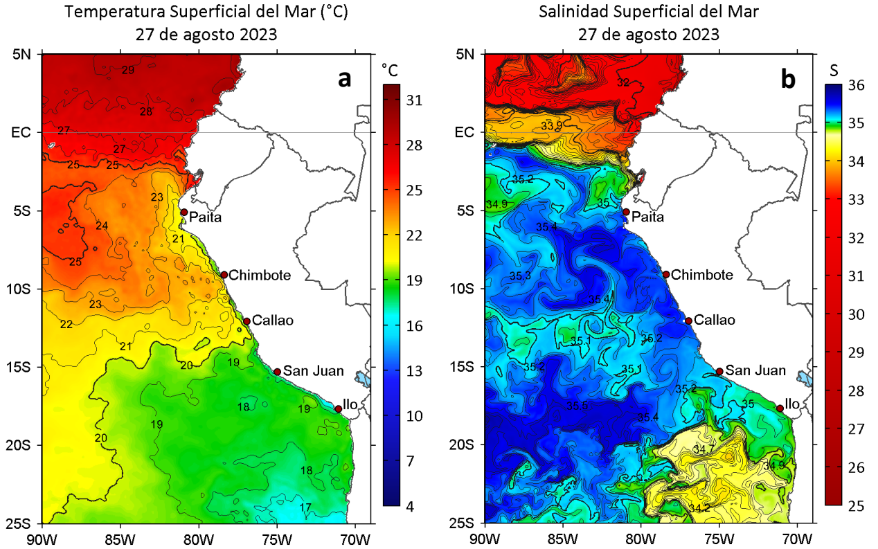
Figura 2. a) Temperatura superficial del mar ( ^{\circ}\text{C} ) y b) Salinidad superficial del mar para el 27 de agosto de 2023. Datos: OSTIA-UKMO-L4-GLOB-v2.0 (UK Met Office, 2012; Donlon et al, 2012) y del GLOBAL_ANALYSISFORECAST_PHY_001_024 (Lellouche, J. M. et al, 2013), respectivamente.
