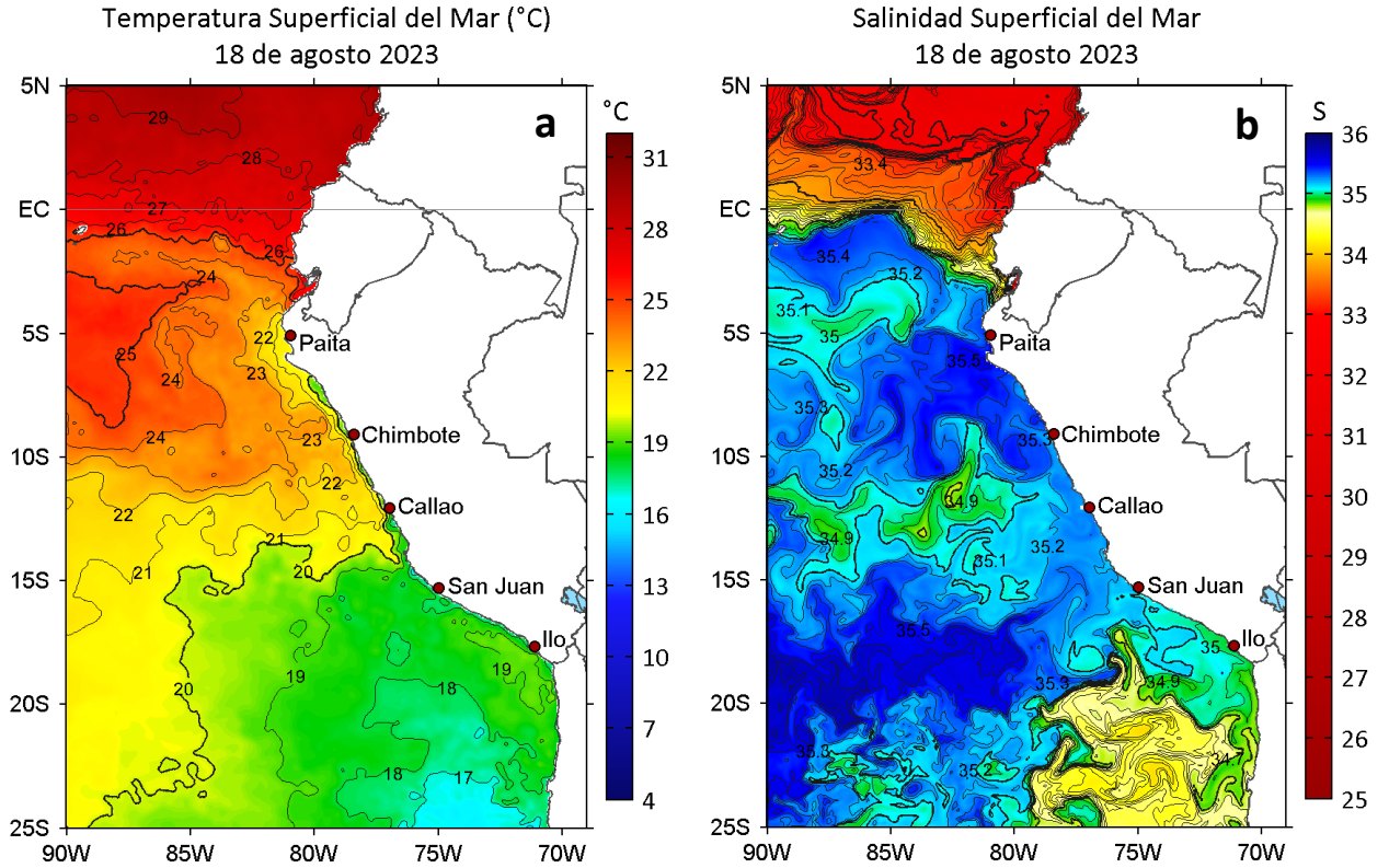
Figura 2. a) Temperatura superficial del mar ( ^{\circ}\text{C} ) y b) Salinidad superficial del mar para el 18 de agosto de 2023. Datos: OSTIA-UKMO-L4-GLOB-v2.0 (UK Met Office, 2012; Donlon et al, 2012) y del GLOBAL_ANALYSISFORECAST_PHY_001_024 (Lellouche, J. M. et al, 2013), respectivamente.
