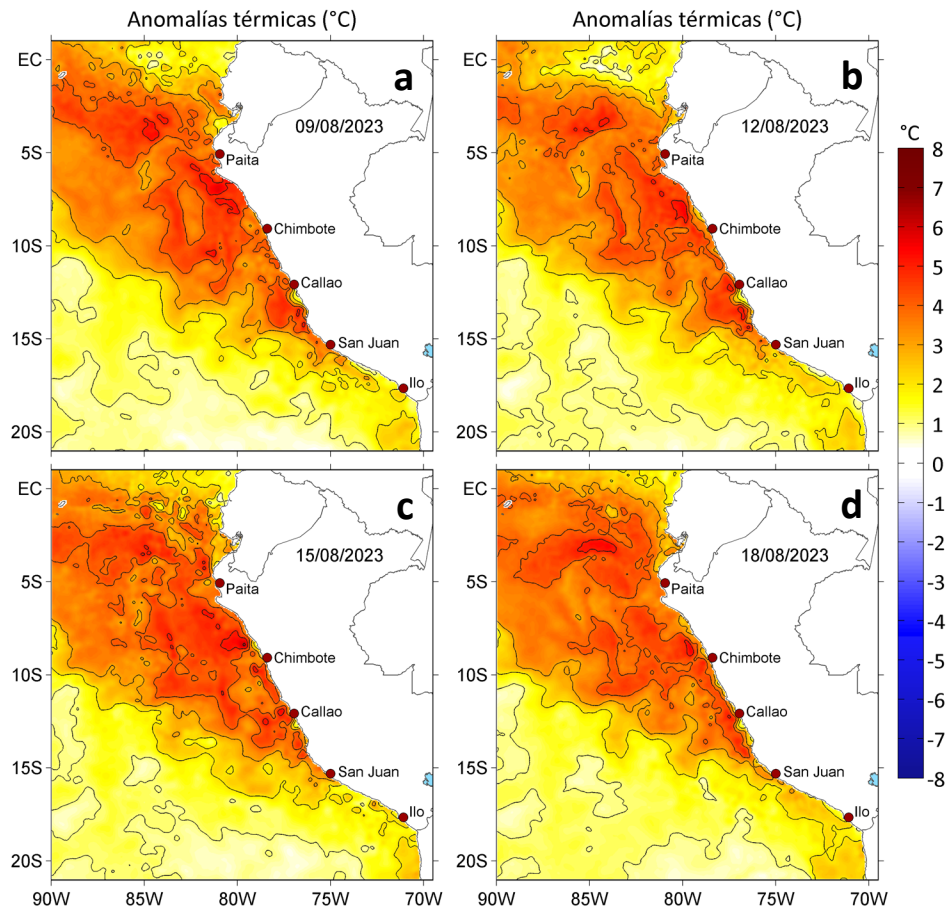
Figura 3. Anomalías de la temperatura superficial del mar ( ^{\circ}\text{C} ) para el a) 09, b) 12, c) 15 y d) 18 de agosto de 2023. Las anomalías se calcularon respecto de la climatología para el periodo 1991-2020. Datos: OSTIA-UKMO-L4-GLOB-v2.0 (UK Met Office, 2012; Donlon et al, 2012).
