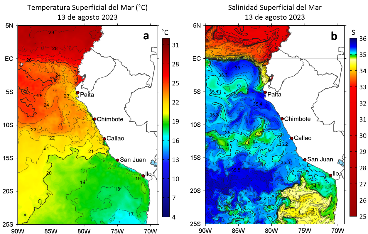
Figura 2. a) Temperatura superficial del mar ( ^{\circ}\text{C} ) y b) Salinidad superficial del mar para el 13 de agosto de 2023. Datos: OSTIA-UKMO-L4-GLOB-v2.0 (UK Met Office, 2012; Donlon et al, 2012) y del GLOBAL_ANALYSISFORECAST_PHY_001_024 (Lellouche, J. M. et al, 2013), respectivamente.
