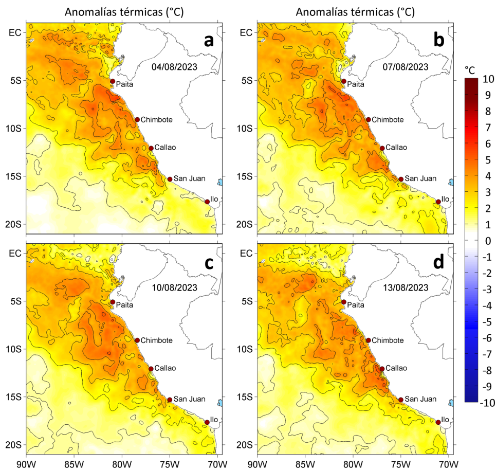
Figura 3. Anomalías de la temperatura superficial del mar ( ^{\circ}\text{C} ) para el a) 04, b) 07, c) 10 y d) 13 de agosto de 2023. Las anomalías se calcularon respecto de la climatología para el periodo 2007-2016. Datos: OSTIA-UKMO-L4-GLOB-v2.0 (UK Met Office, 2012; Donlon et al, 2012).
