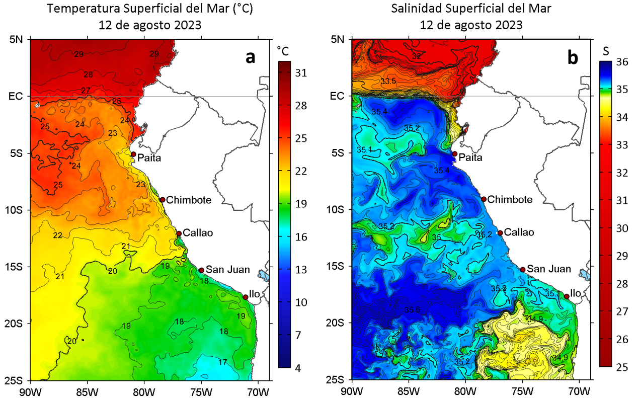
Figura 2. a) Temperatura superficial del mar ( ^{\circ}\text{C} ) y b) Salinidad superficial del mar para el 12 de agosto de 2023. Datos: OSTIA-UKMO-L4-GLOB-v2.0 (UK Met Office, 2012; Donlon et al, 2012) y del GLOBAL_ANALYSISFORECAST_PHY_001_024 (Lellouche, J. M. et al, 2013), respectivamente.
