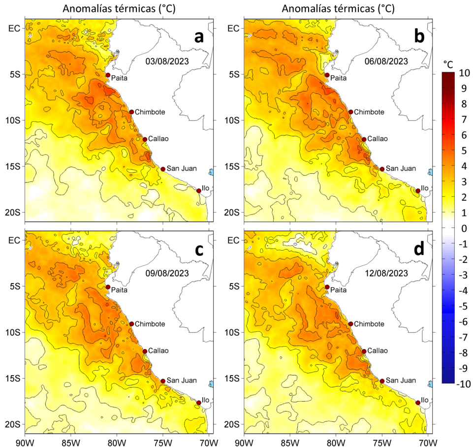
Figura 3. Anomalías de la temperatura superficial del mar ( ^{\circ}\text{C} ) para el a) 03, b) 06, c) 09 y d) 12 de agosto de 2023. Las anomalías se calcularon respecto de la climatología para el periodo 2007-2016. Datos: OSTIA-UKMO-L4-GLOB-v2.0 (UK Met Office, 2012; Donlon et al, 2012).
