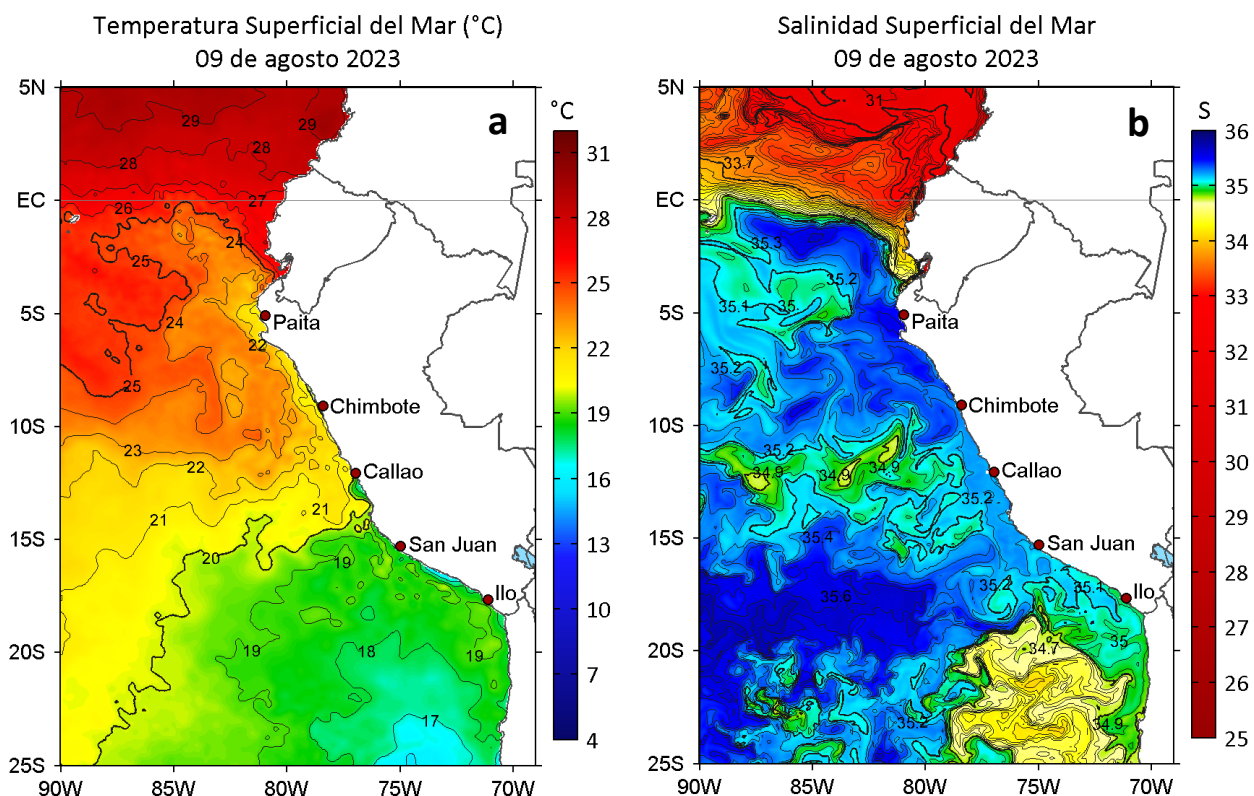
Figura 2. a) Temperatura superficial del mar ( ^{\circ}\text{C} ) y b) Salinidad superficial del mar para el 09 de agosto de 2023. Datos: OSTIA-UKMO-L4-GLOB-v2.0 (UK Met Office, 2012; Donlon et al, 2012) y del GLOBAL_ANALYSISFORECAST_PHY_001_024 (Lellouche, J. M. et al, 2013), respectivamente.
