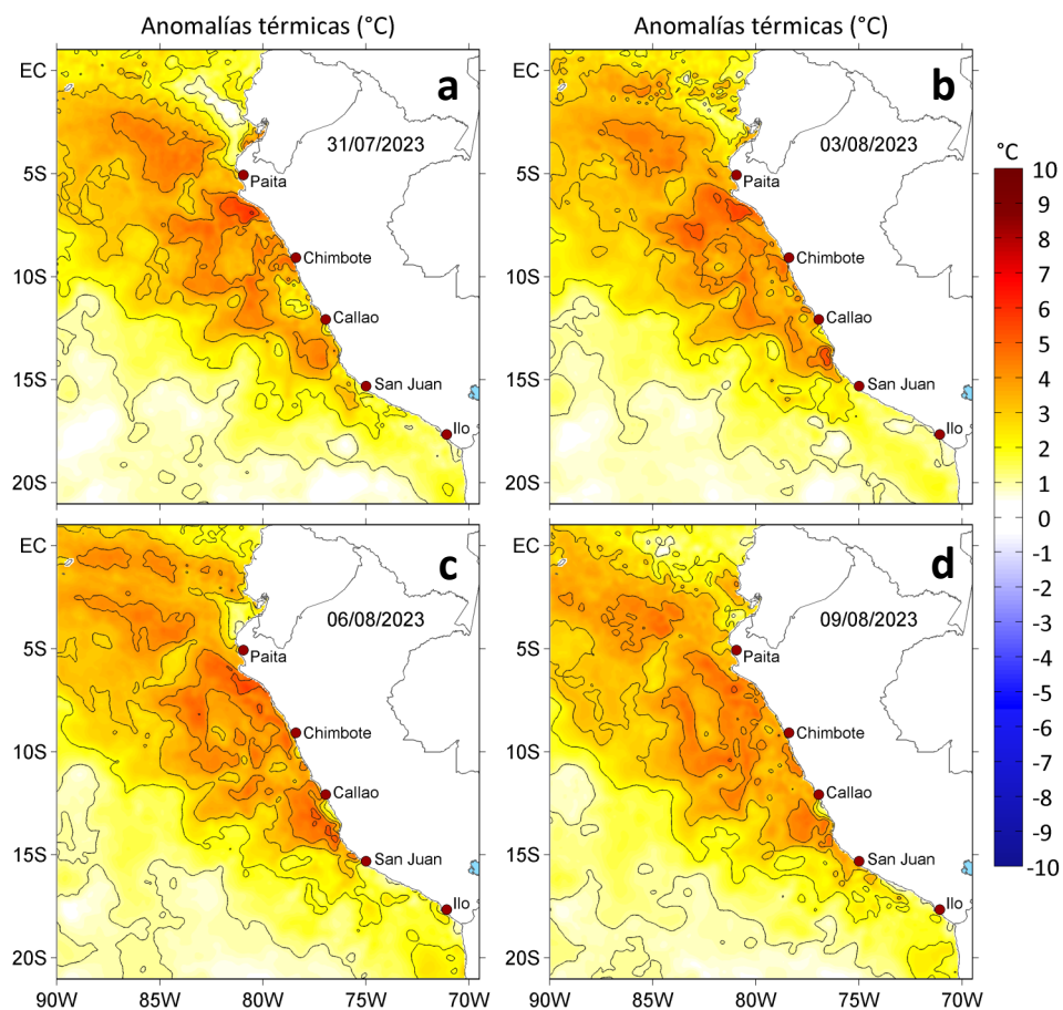
Figura 3. Anomalías de la temperatura superficial del mar ( ^{\circ}\text{C} ) para el a) 31 de julio, b) 03, c) 06 y d) 09 de agosto de 2023. Las anomalías se calcularon respecto de la climatología para el periodo 2007-2016. Datos: OSTIA-UKMO-L4-GLOB-v2.0 (UK Met Office, 2012; Donlon et al, 2012).
