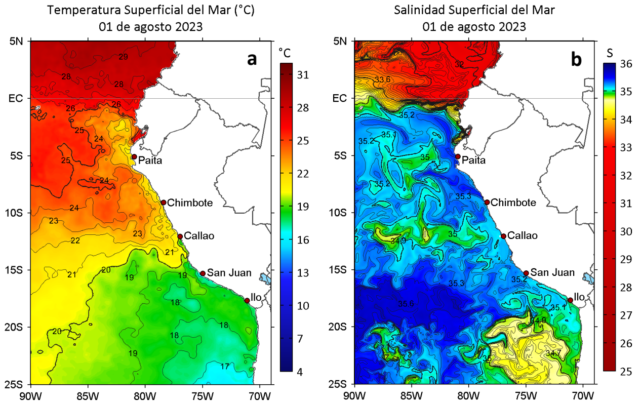
Figura 2. a) Temperatura superficial del mar ( ^{\circ}\text{C} ) y b) Salinidad superficial del mar para el 01 de agosto de 2023. Datos: OSTIA-UKMO-L4-GLOB-v2.0 (UK Met Office, 2012; Donlon et al, 2012) y del GLOBAL_ANALYSISFORECAST_PHY_001_024 (Lellouche, J. M. et al, 2013), respectivamente.
