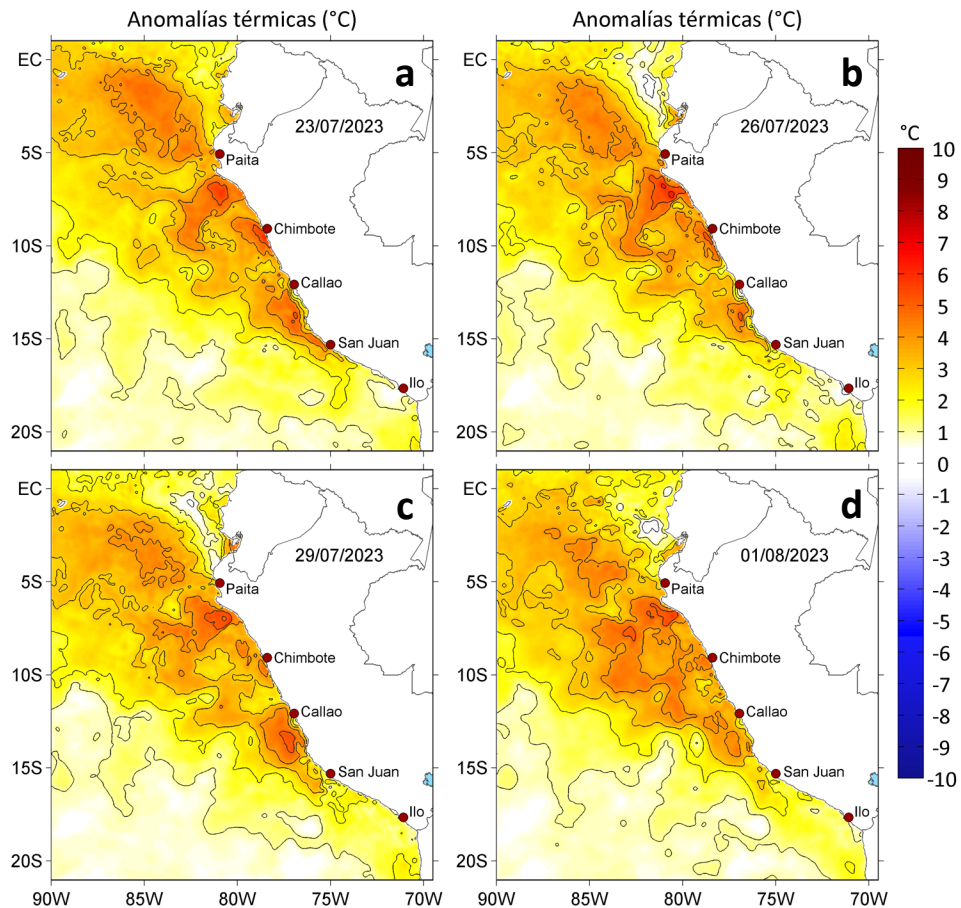
Figura 3. Anomalías de la temperatura superficial del mar ( ^{\circ}\text{C} ) para el a) 23, b) 26 y c) 29 de julio, así como para d) 01 de agosto de 2023. Las anomalías se calcularon respecto de la climatología para el periodo 2007-2016. Datos: OSTIA-UKMO-L4-GLOB-v2.0 (UK Met Office, 2012; Donlon et al, 2012).
