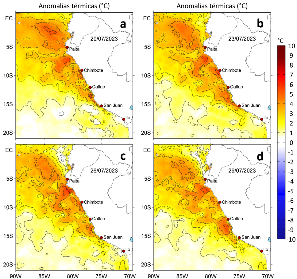
Figura 3. Anomalías de la temperatura superficial del mar ( ^{\circ}\text{C} ) para el a) 20, b) 23, c) 26 y d) 29 de julio de 2023. Las anomalías se calcularon respecto de la climatología para el periodo 2007-2016. Datos: OSTIA-UKMO-L4-GLOB-v2.0 (UK Met Office, 2012; Donlon et al, 2012).
