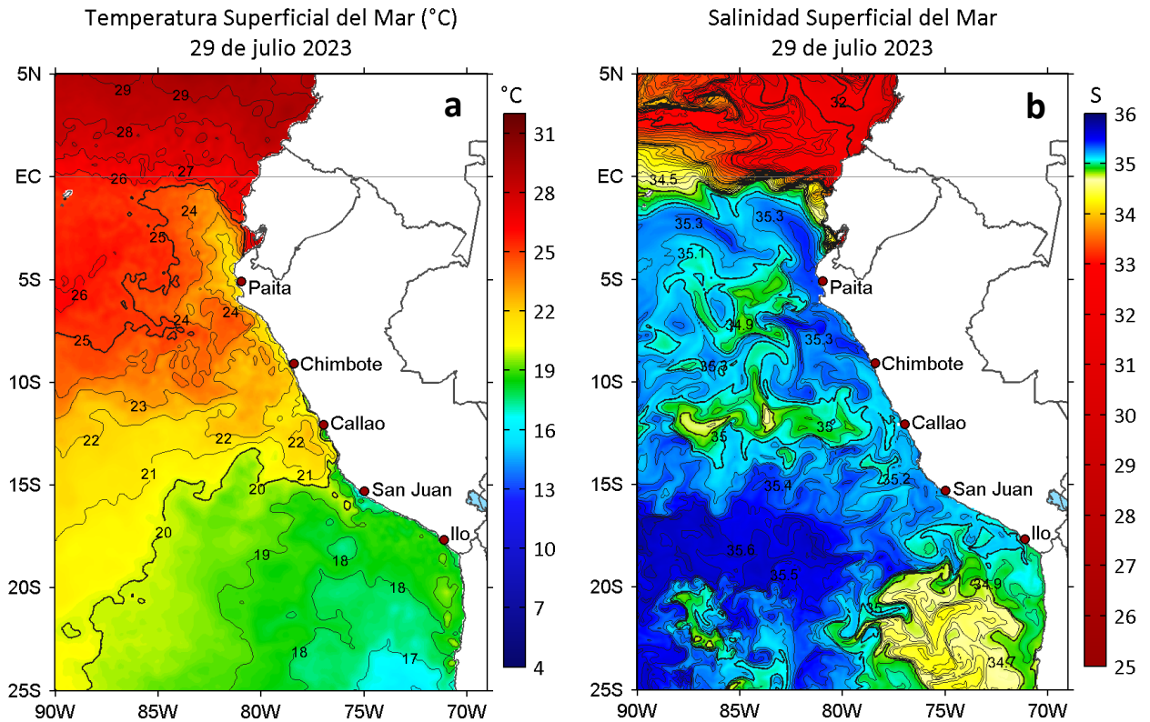
Figura 2. a) Temperatura superficial del mar ( ^{\circ}\text{C} ) y b) Salinidad superficial del mar para el 29 de julio de 2023. Datos: OSTIA-UKMO-L4-GLOB-v2.0 (UK Met Office, 2012; Donlon et al, 2012) y del GLOBAL_ANALYSISFORECAST_PHY_001_024 (Lellouche, J. M. et al, 2013), respectivamente.
