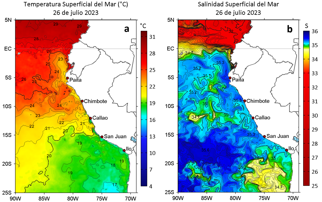
Figura 2. a) Temperatura superficial del mar ( ^{\circ}\text{C} ) y b) Salinidad superficial del mar para el 26 de julio de 2023. Datos: OSTIA-UKMO-L4-GLOB-v2.0 (UK Met Office, 2012; Donlon et al, 2012) y del GLOBAL_ANALYSISFORECAST_PHY_001_024 (Lellouche, J. M. et al, 2013), respectivamente.
