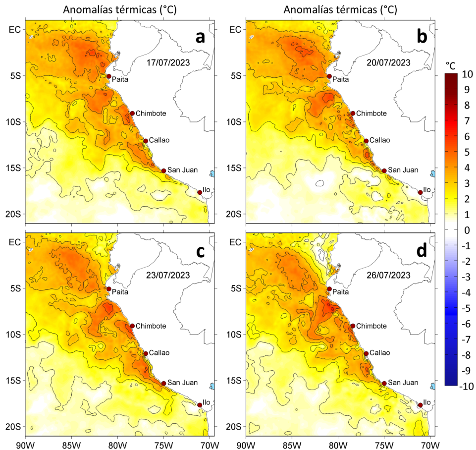
Figura 3. Anomalías de la temperatura superficial del mar ( ^{\circ}\text{C} ) para el a) 17, b) 20, c) 23 y d) 26 de julio de 2023. Las anomalías se calcularon respecto de la climatología para el periodo 2007-2016. Datos: OSTIA-UKMO-L4-GLOB-v2.0 (UK Met Office, 2012; Donlon et al, 2012).
