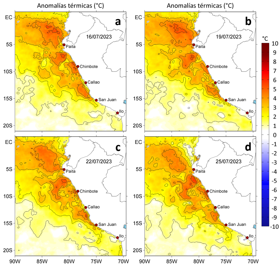
Figura 3. Anomalías de la temperatura superficial del mar ( ^{\circ}\text{C} ) para el a) 16, b) 19, c) 22 y d) 25 de julio de 2023. Las anomalías se calcularon respecto de la climatología para el periodo 2007-2016. Datos: OSTIA-UKMO-L4-GLOB-v2.0 (UK Met Office, 2012; Donlon et al, 2012).
