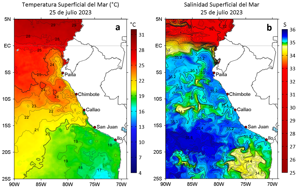
Figura 2. a) Temperatura superficial del mar ( ^{\circ}\text{C} ) y b) Salinidad superficial del mar para el 25 de julio de 2023. Datos: OSTIA-UKMO-L4-GLOB-v2.0 (UK Met Office, 2012; Donlon et al, 2012) y del GLOBAL_ANALYSISFORECAST_PHY_001_024 (Lellouche, J. M. et al, 2013), respectivamente.
