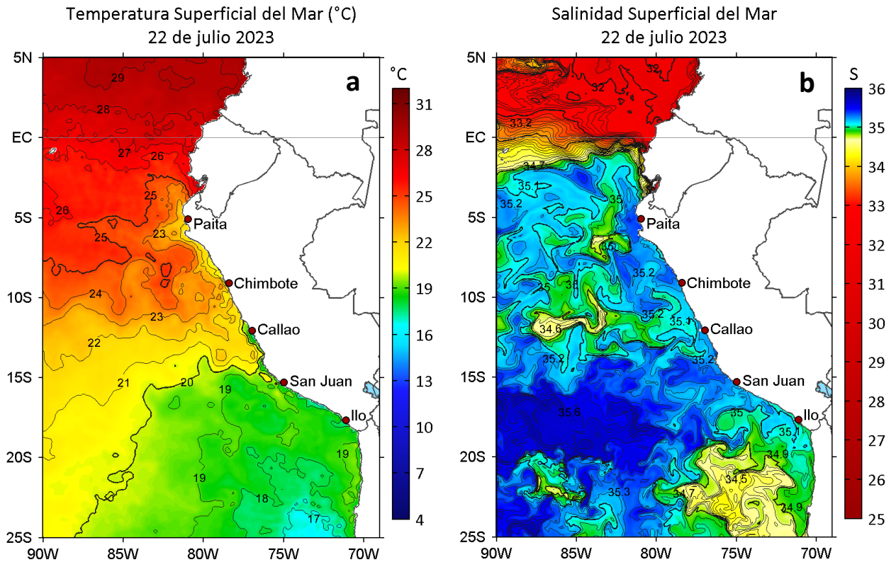
Figura 2. a) Temperatura superficial del mar ( ^{\circ}\text{C} ) y b) Salinidad superficial del mar para el 22 de julio de 2023. Datos: OSTIA-UKMO-L4-GLOB-v2.0 (UK Met Office, 2012; Donlon et al, 2012) y del GLOBAL_ANALYSISFORECAST_PHY_001_024 (Lellouche, J. M. et al, 2013), respectivamente.
