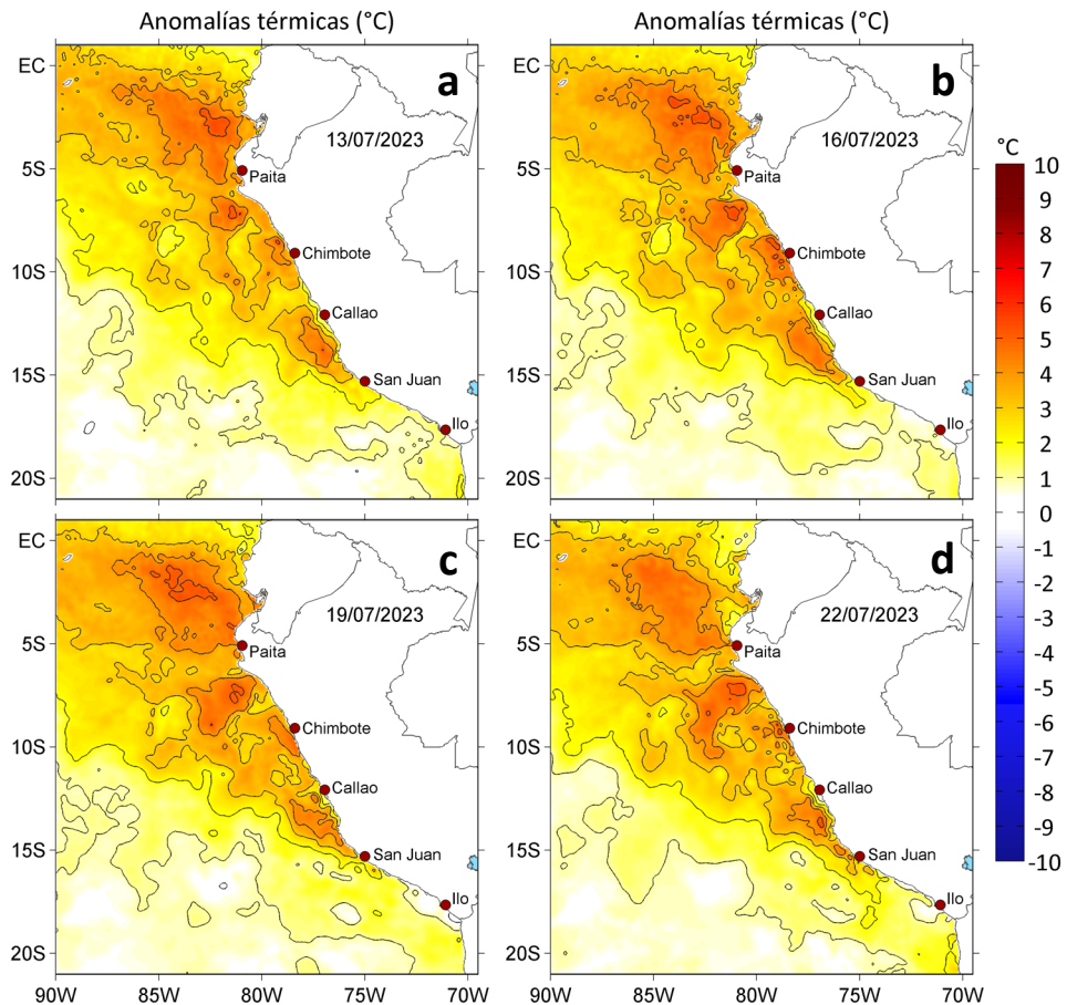
Figura 3. Anomalías de la temperatura superficial del mar ( ^{\circ}\text{C} ) para el a) 13, b) 16, c) 19 y d) 22 de julio de 2023. Las anomalías se calcularon respecto de la climatología para el periodo 2007-2016. Datos: OSTIA-UKMO-L4-GLOB-v2.0 (UK Met Office, 2012; Donlon et al, 2012).
