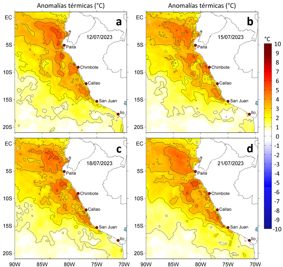
Figura 3. Anomalías de la temperatura superficial del mar ( ^{\circ}\text{C} ) para el a) 12, b) 15, c) 18 y d) 21 de julio de 2023. Las anomalías se calcularon respecto de la climatología para el periodo 2007-2016. Datos: OSTIA-UKMO-L4-GLOB-v2.0 (UK Met Office, 2012; Donlon et al, 2012).
