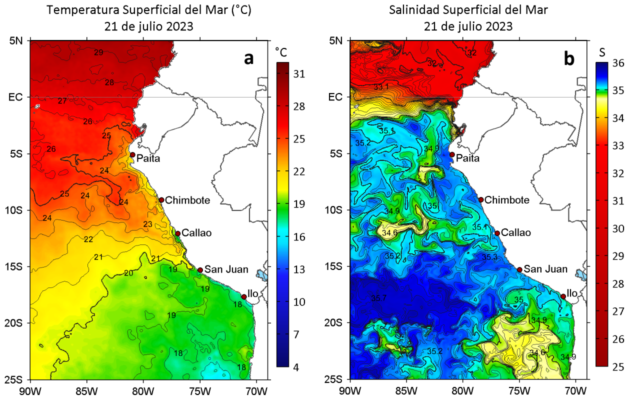
Figura 2. a) Temperatura superficial del mar ( ^{\circ}\text{C} ) y b) Salinidad superficial del mar para el 21 de julio de 2023. Datos: OSTIA-UKMO-L4-GLOB-v2.0 (UK Met Office, 2012; Donlon et al, 2012) y del GLOBAL_ANALYSISFORECAST_PHY_001_024 (Lellouche, J. M. et al, 2013), respectivamente.
