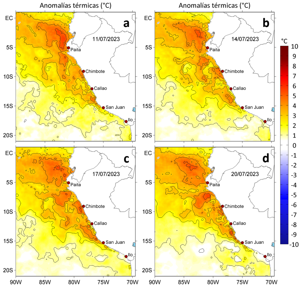
Figura 3. Anomalías de la temperatura superficial del mar ( ^{\circ}\text{C} ) para el a) 11, b) 14, c) 17 y d) 20 de julio de 2023. Las anomalías se calcularon respecto de la climatología para el periodo 2007-2016. Datos: OSTIA-UKMO-L4-GLOB-v2.0 (UK Met Office, 2012; Donlon et al, 2012).
