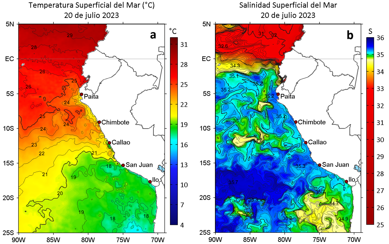
Figura 2. a) Temperatura superficial del mar ( ^{\circ}\text{C} ) y b) Salinidad superficial del mar para el 20 de julio de 2023. Datos: OSTIA-UKMO-L4-GLOB-v2.0 (UK Met Office, 2012; Donlon et al, 2012) y del GLOBAL_ANALYSISFORECAST_PHY_001_024 (Lellouche, J. M. et al, 2013), respectivamente.
