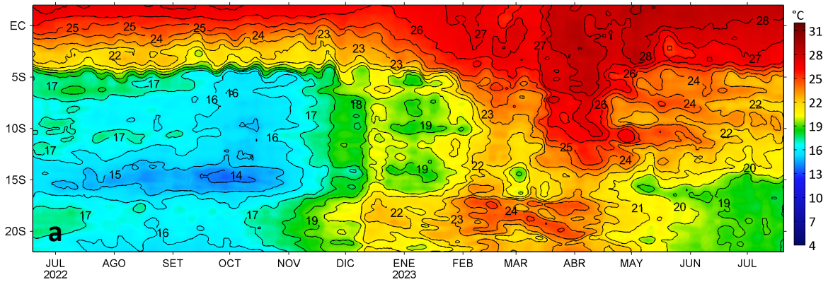
Anomalías de la Temperatura Superficial del mar (°C), franja costera de 60 m.n. 19 de junio 2022 - 20 de julio 2023
