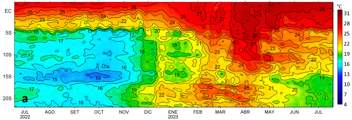
Anomalías de la Temperatura Superficial del mar (°C), franja costera de 60 m.n. 18 de junio 2022 - 19 de julio 2023
