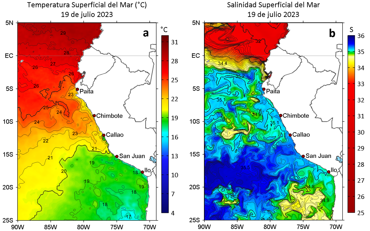
Figura 2. a) Temperatura superficial del mar ( ^{\circ}\text{C} ) y b) Salinidad superficial del mar para el 19 de julio de 2023. Datos: OSTIA-UKMO-L4-GLOB-v2.0 (UK Met Office, 2012; Donlon et al, 2012) y del GLOBAL_ANALYSISFORECAST_PHY_001_024 (Lellouche, J. M. et al, 2013), respectivamente.
