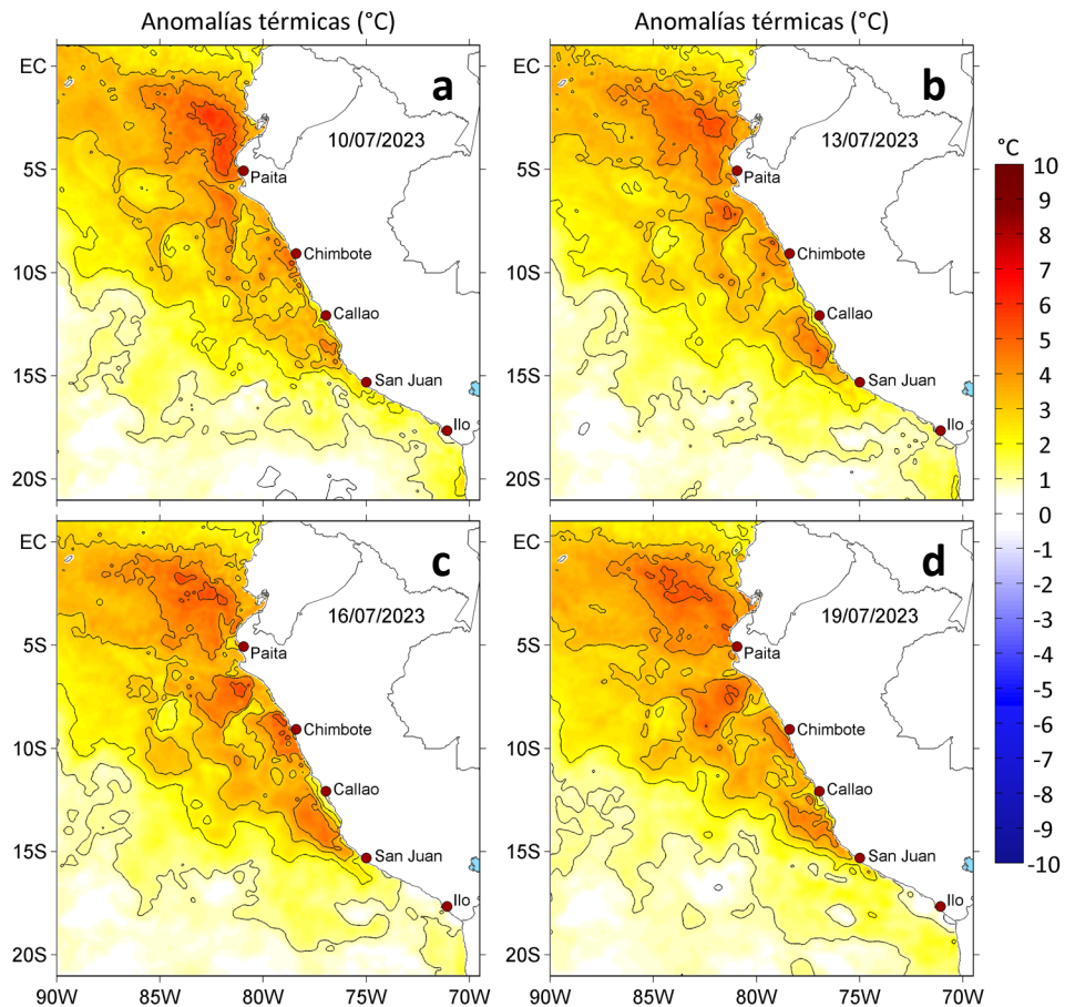
Figura 3. Anomalías de la temperatura superficial del mar ( ^{\circ}\text{C} ) para el a) 10, b) 13, c) 16 y d) 19 de julio de 2023. Las anomalías se calcularon respecto de la climatología para el periodo 2007-2016. Datos: OSTIA-UKMO-L4-GLOB-v2.0 (UK Met Office, 2012; Donlon et al, 2012).
