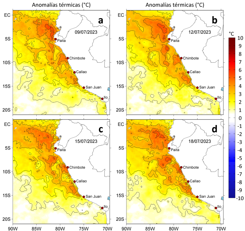
Figura 3. Anomalías de la temperatura superficial del mar ( ^{\circ}\text{C} ) para el a) 09, b) 12, c) 15 y d) 18 de julio de 2023. Las anomalías se calcularon respecto de la climatología para el periodo 2007-2016. Datos: OSTIA-UKMO-L4-GLOB-v2.0 (UK Met Office, 2012; Donlon et al, 2012).
