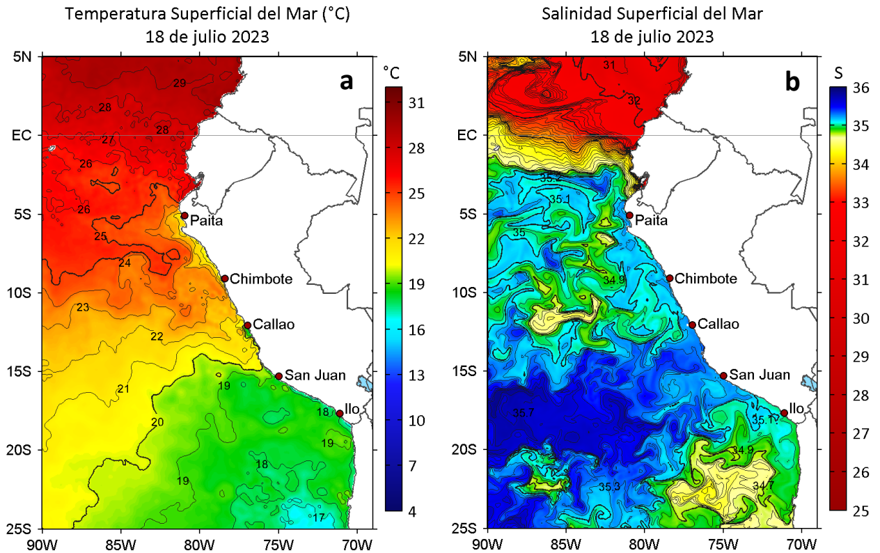
Figura 2. a) Temperatura superficial del mar ( ^{\circ}\text{C} ) y b) Salinidad superficial del mar para el 18 de julio de 2023. Datos: OSTIA-UKMO-L4-GLOB-v2.0 (UK Met Office, 2012; Donlon et al, 2012) y del GLOBAL_ANALYSISFORECAST_PHY_001_024 (Lellouche, J. M. et al, 2013), respectivamente.
